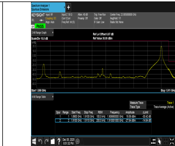
Band2-20MHz-QPSK-19100-1RB#99-PASS
