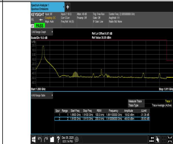
Band2-20MHz-16QAM-19100-1RB#0-PASS
