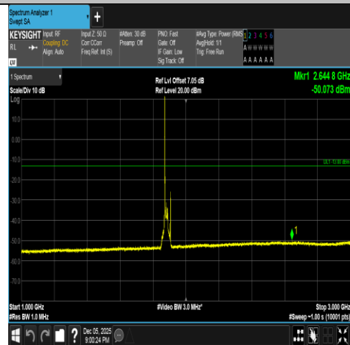
Band2-20MHz-QPSK-18900-1RB#0-1000~3000-PASS
