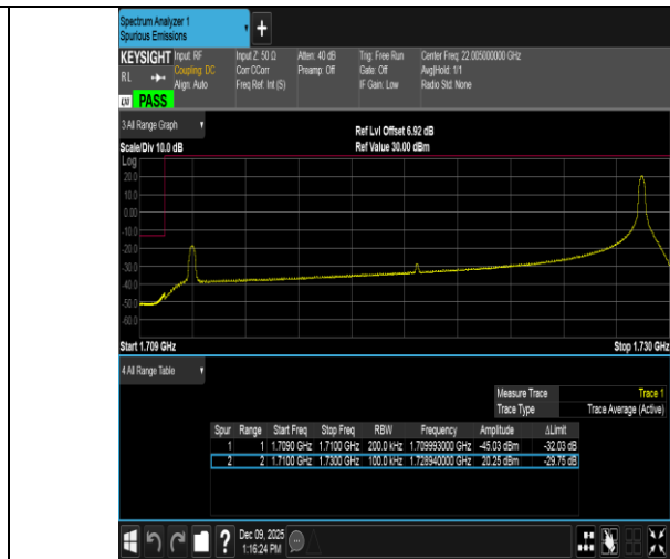
Band4-20MHz-QPSK-20050-1RB#99-PASS
