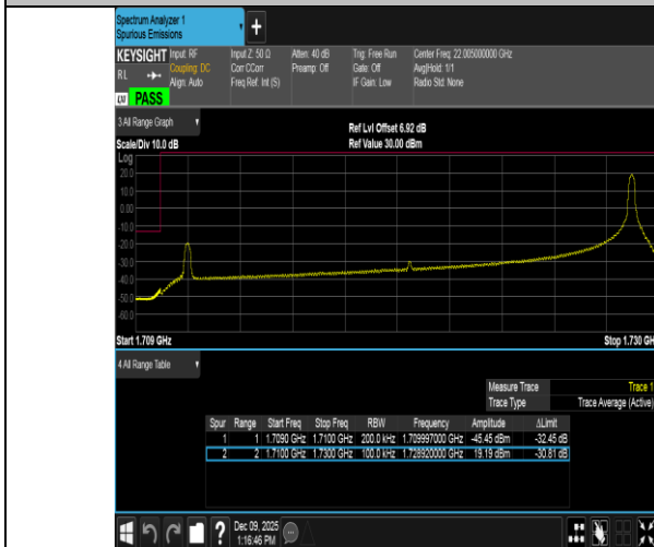
Band4-20MHz-16QAM-20050-1RB#99-PASS
