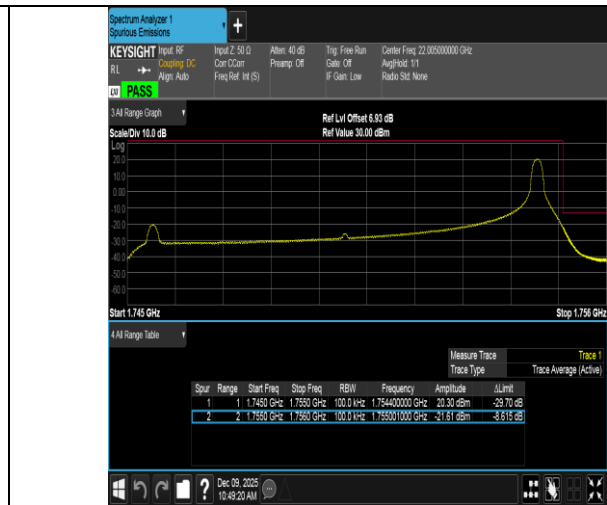
Band4-10MHz-QPSK-20350-1RB#49-PASS
