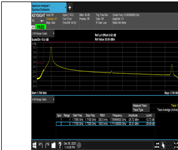
Band4-20MHz-QPSK-20050-1RB#0-PASS
