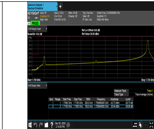
Band66-20MHz-QPSK-132072-1RB#99-PASS
