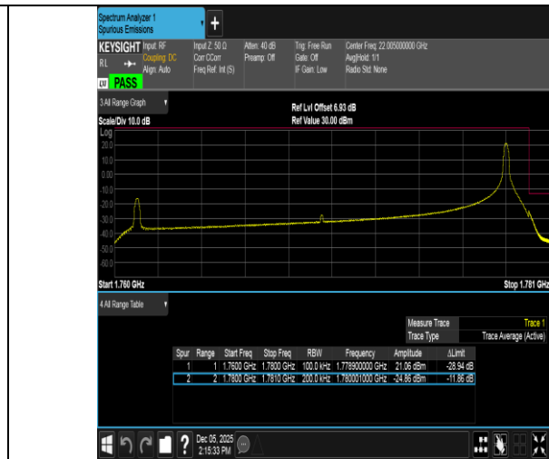
Band66-20MHz-QPSK-132572-1RB#99-PASS
