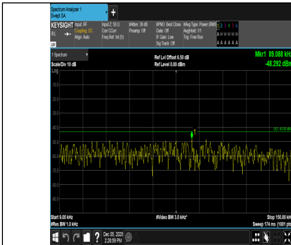
Band66-20MHz-QPSK-132572-1RB#0-0.009~0.15-PASS
