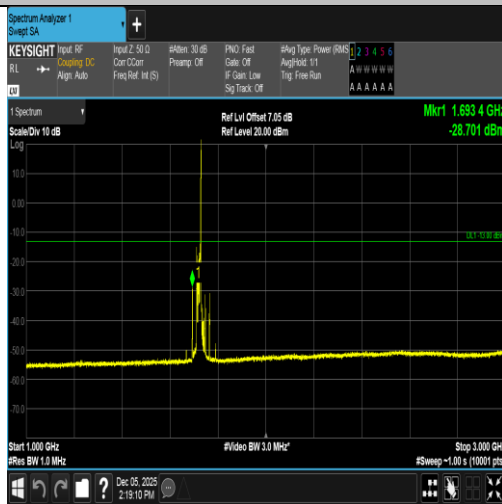
Band66-20MHz-QPSK-132072-1RB#99-1000~3000-PASS
