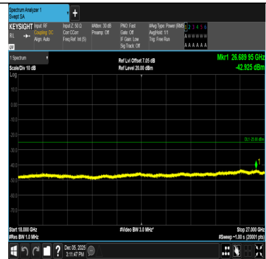
Band7-15MHz-QPSK-20825-1RB#0-18000~27000-PASS
