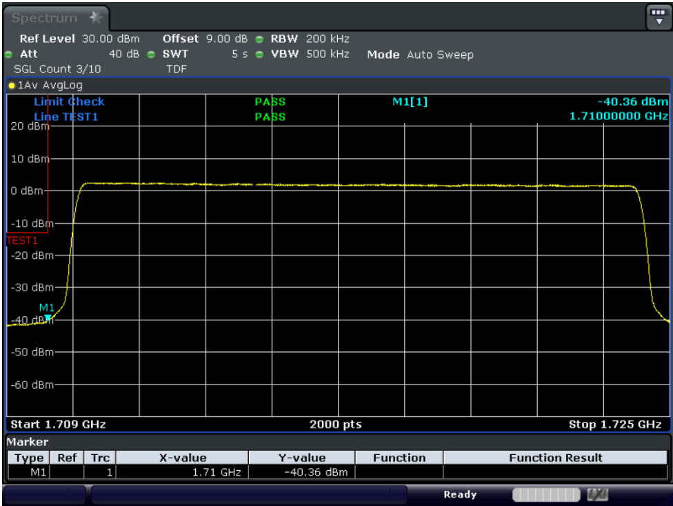
Test_Graph_band66_1717.5MHz_15M_QPSK_75RB#LOW_Band edge
