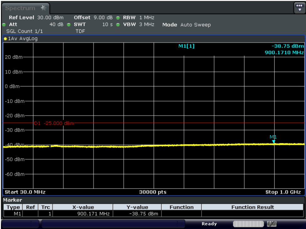
Test_Graph_band7_2562.5MHz_15M_QPSK_75RB#LOW_30M_1G_TX
