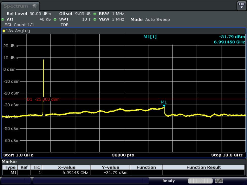
Test_Graph_band7_2535MHz_15M_QPSK_75RB#LOW_1G_10G_TX
