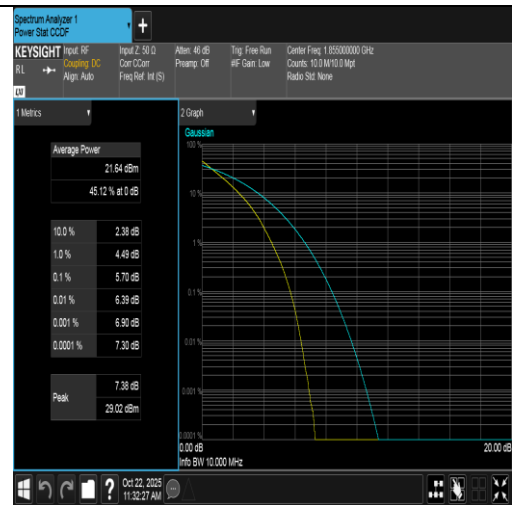
Band2-10MHz-QPSK-18650-50RB#0-PASS
