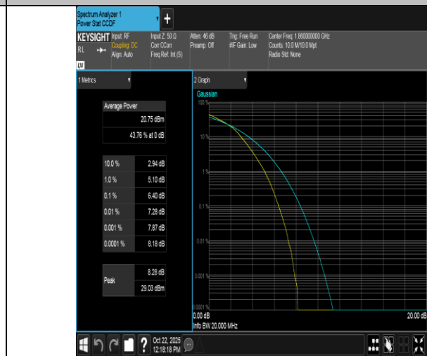
Band2-20MHz-16QAM-18700-100RB#0-PASS
