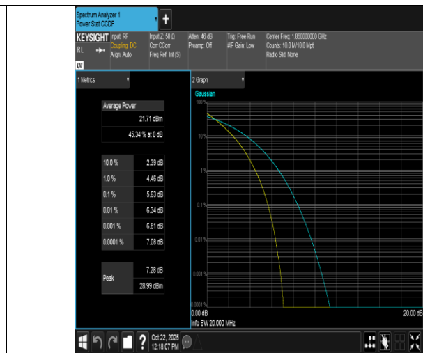
Band2-20MHz-QPSK-18700-100RB#0-PASS
