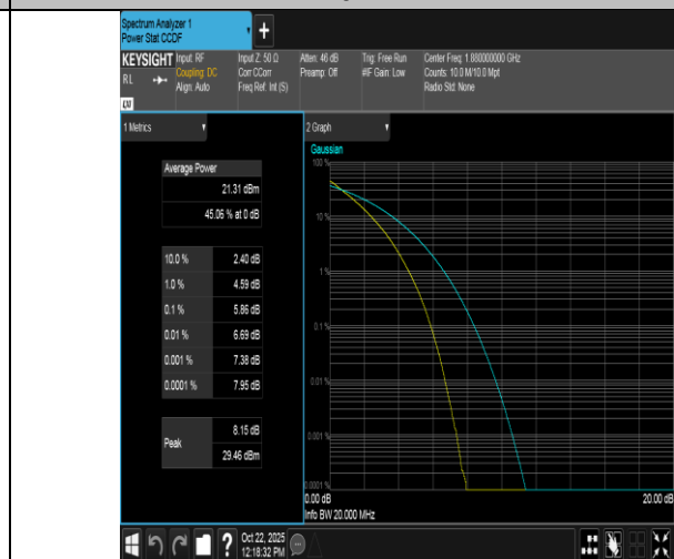
Band2-20MHz-QPSK-18900-100RB#0-PASS
