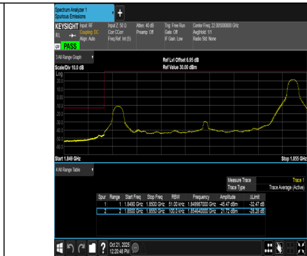
Band2-5MHz-QPSK-18625-1RB#24-PASS
