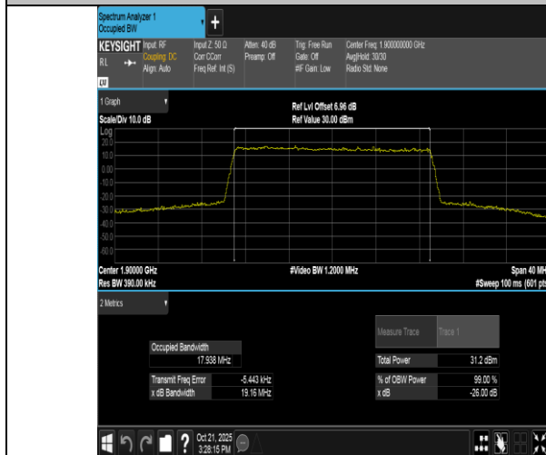
Band2-20MHz-QPSK-19100-100RB#0-PASS
