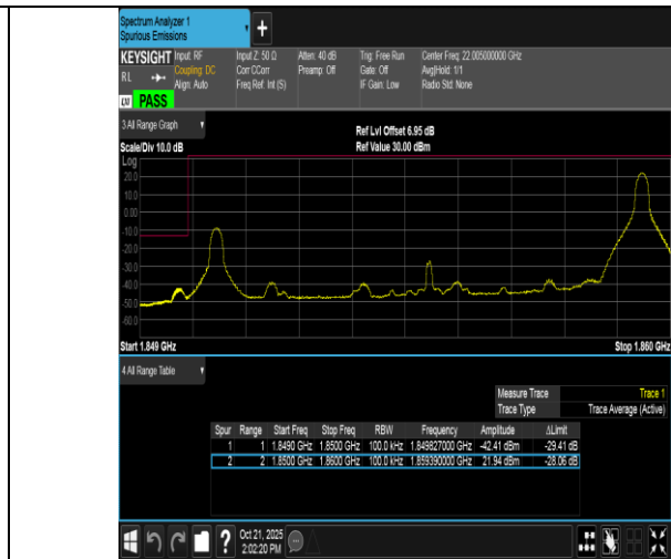
Band2-10MHz-QPSK-18650-1RB#49-PASS
