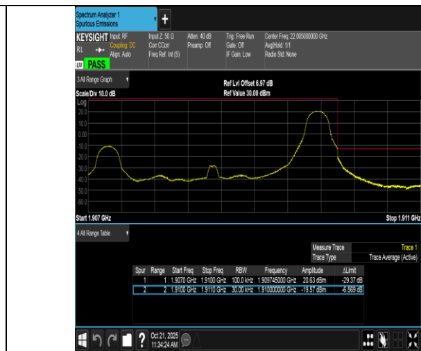
Band2-3MHz-QPSK-19185-1RB#14-PASS
