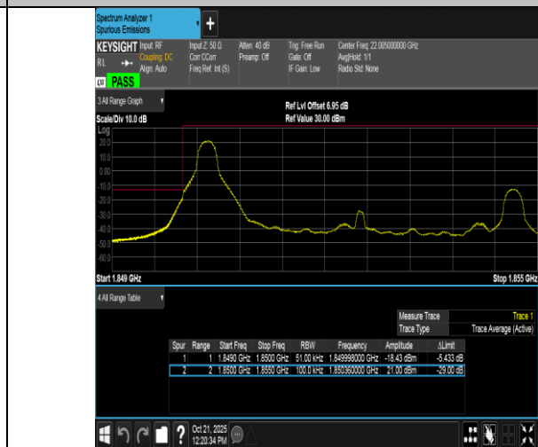
Band2-5MHz-16QAM-18625-1RB#0-PASS
