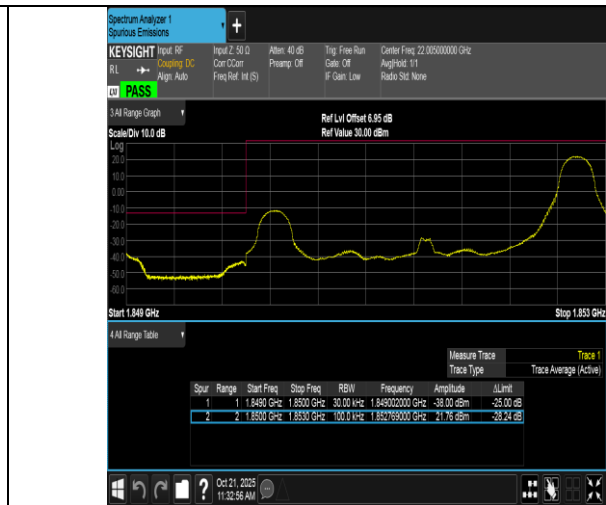
Band2-3MHz-QPSK-18615-1RB#14-PASS
