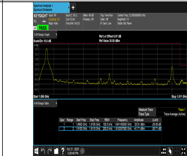
Band2-20MHz-16QAM-19100-1RB#0-PASS
