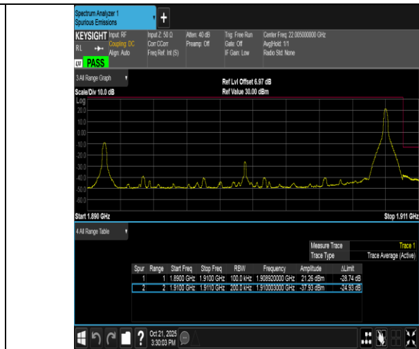
Band2-20MHz-QPSK-19100-1RB#99-PASS
