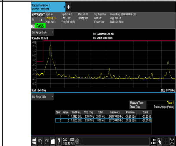
Band2-20MHz-16QAM-18700-1RB#0-PASS
