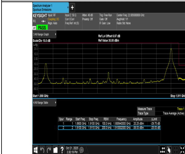
Band2-20MHz-16QAM-19100-1RB#99-PASS
