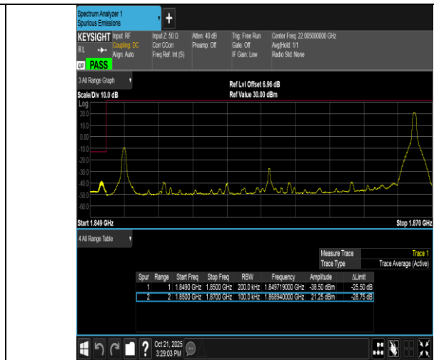
Band2-20MHz-QPSK-18700-1RB#99-PASS
