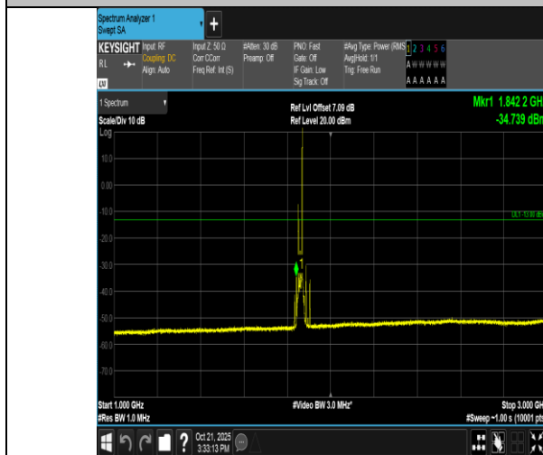
Band2-20MHz-QPSK-18700-1RB#99-1000~3000-PASS
