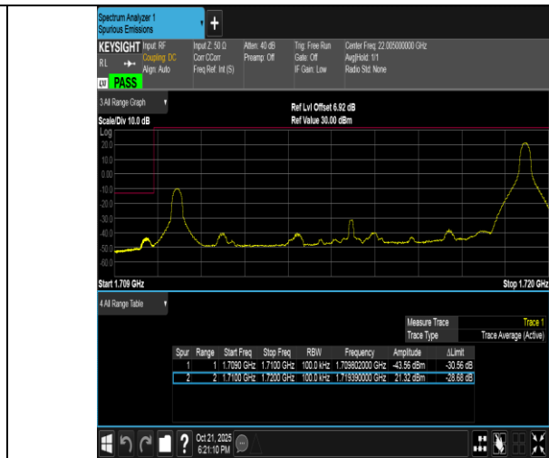
Band4-10MHz-QPSK-20000-1RB#49-PASS
