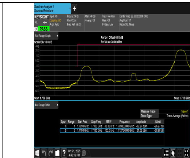
Band4-3MHz-QPSK-19965-1RB#14-PASS
