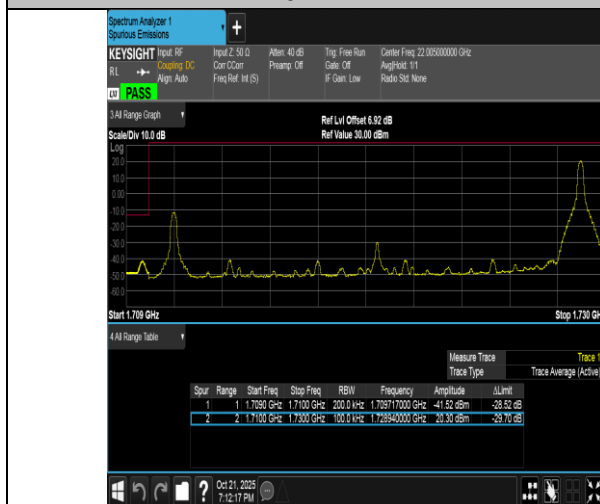
Band4-20MHz-16QAM-20050-1RB#99-PASS
