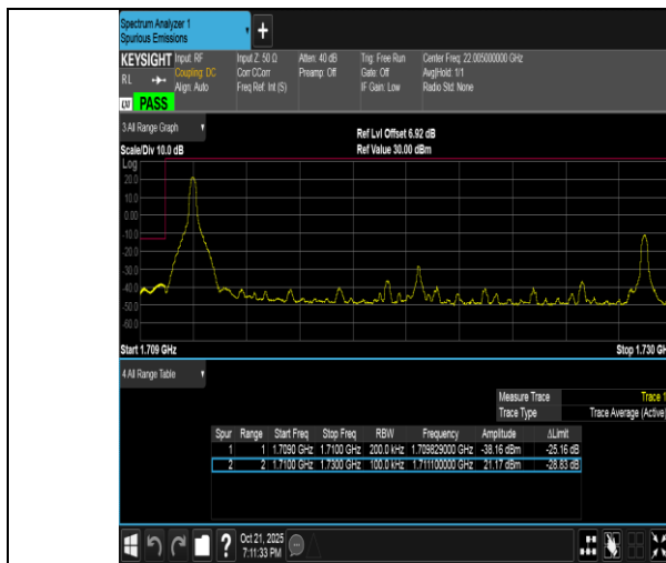
Band4-20MHz-QPSK-20050-1RB#0-PASS
