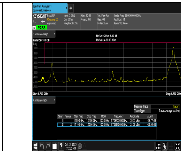
Band4-20MHz-QPSK-20050-1RB#99-PASS
