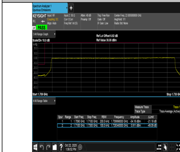
Band4-20MHz-QPSK-20050-100RB#0-PASS
