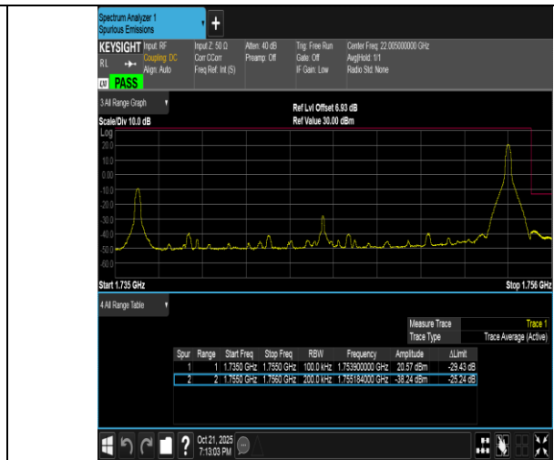
Band4-20MHz-QPSK-20300-1RB#99-PASS
