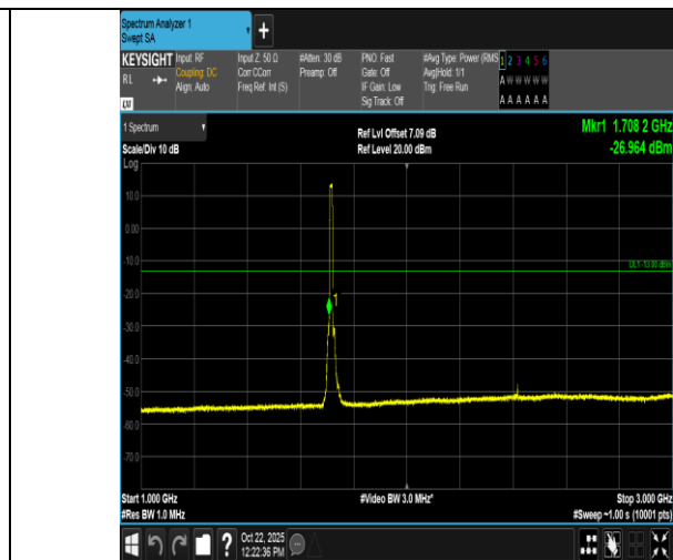
Band4-10MHz-QPSK-20000-50RB#0-1000~3000-PASS
