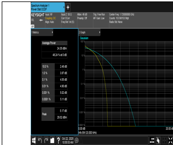
Band66-20MHz-QPSK-132072-1RB#0-PASS
