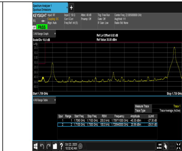
Band66-20MHz-QPSK-132072-1RB#99-PASS
