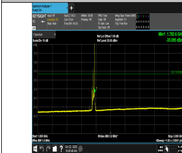
Band66-20MHz-QPSK-132572-1RB#99-1000~3000-PASS
