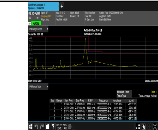
Band7-20MHz-QPSK-21350-1RB#99-PASS
