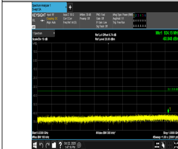
Band7-10MHz-QPSK-20800-50RB#0-30~1000-PASS
