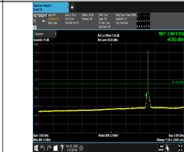
Band7-10MHz-QPSK-20800-50RB#0-1000~3000-PASS
