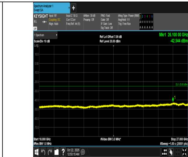
Band7-20MHz-QPSK-20850-1RB#99-18000~27000-PASS
