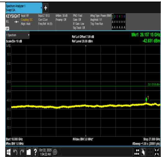
Band7-20MHz-QPSK-21350-1RB#99-18000~27000-PASS
