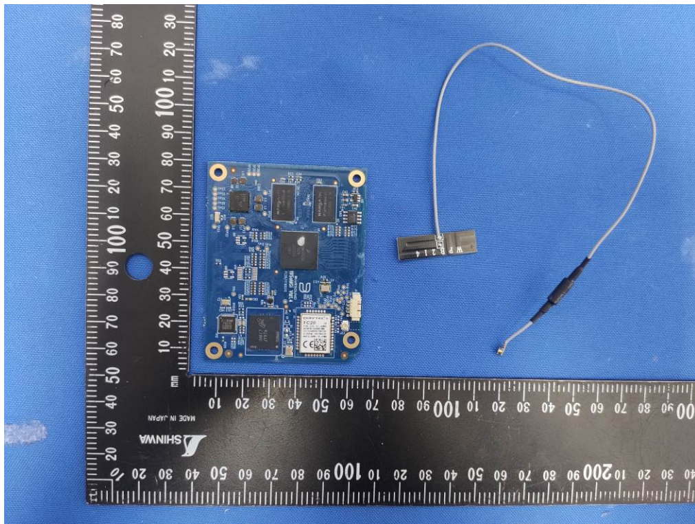
(37) EUT Photo
