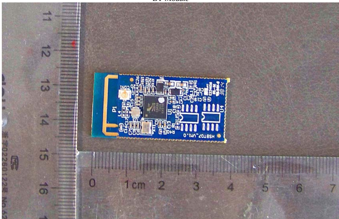
BT Module
