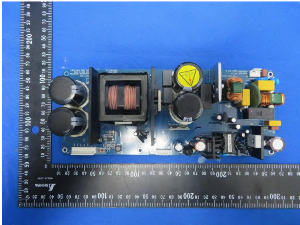
(47) EUT Photo
