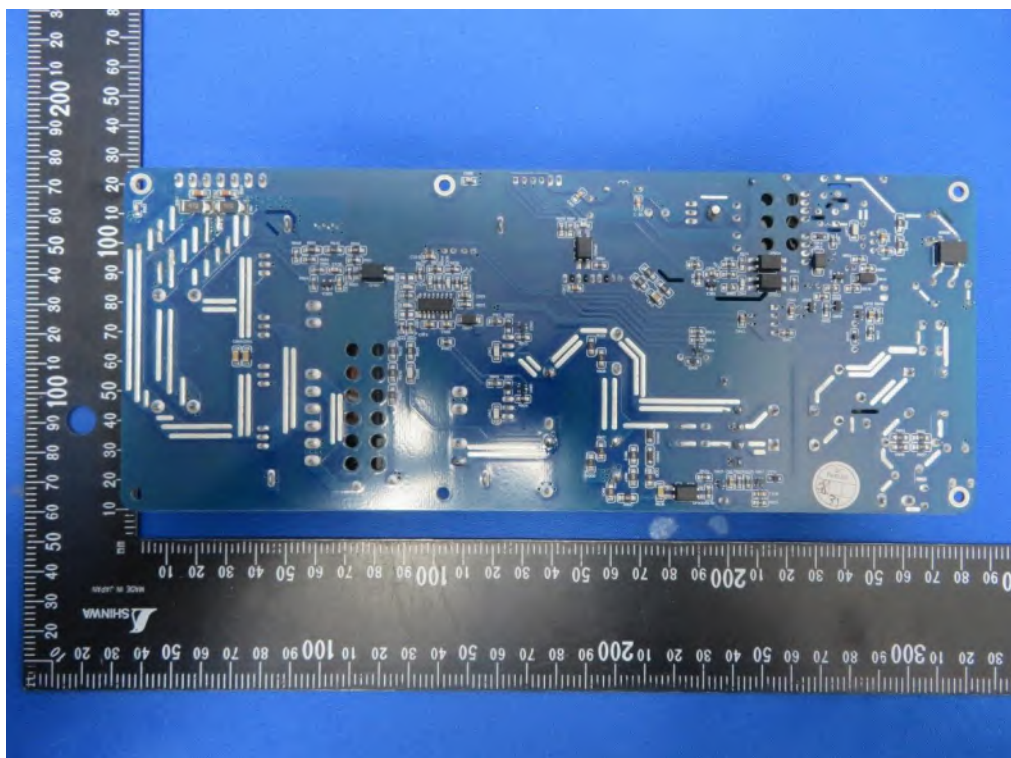
(48) EUT Photo
