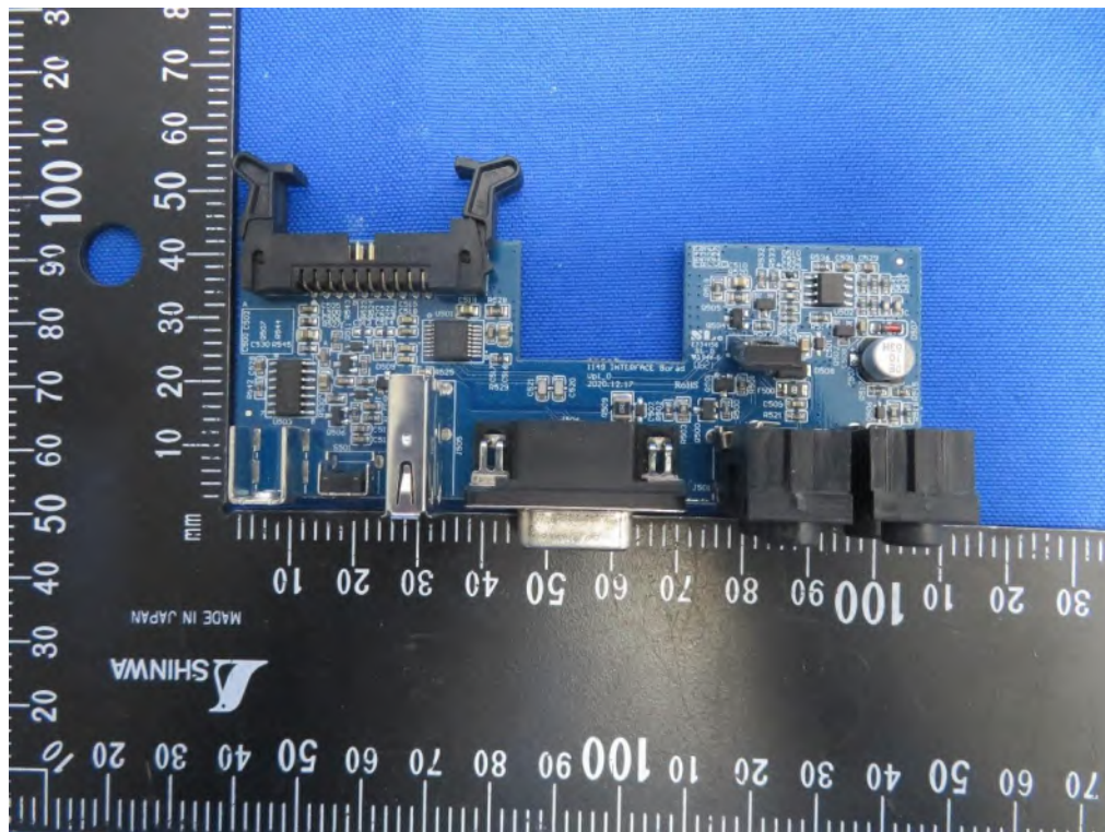
(6) EUT Photo
