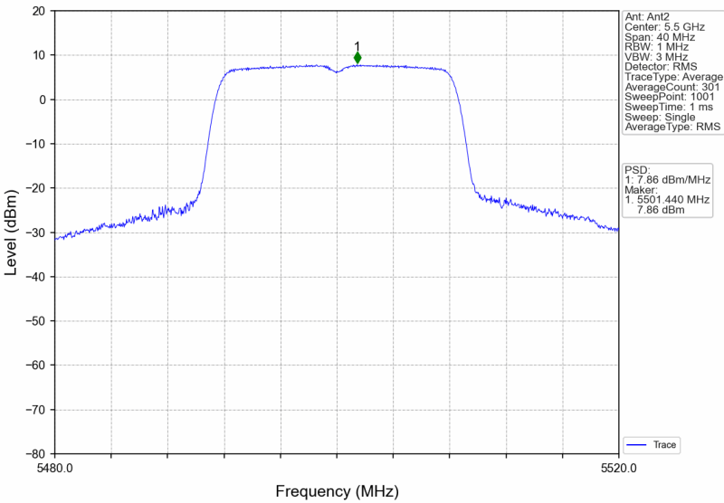
802.11a_MCH_5580MHz_Ant1_NTNV
