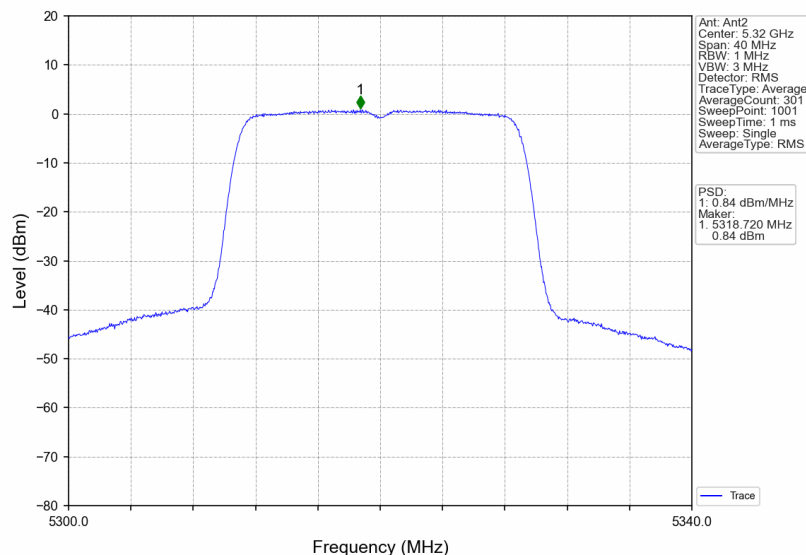
802.11n(HT20)_HCH_5320MHz_MIMO_NTNV
