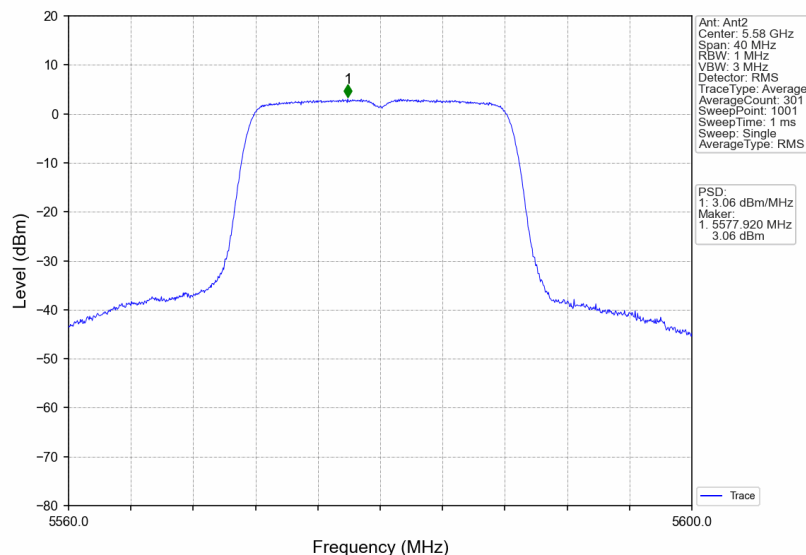
802.11n(HT20)_MCH_5580MHz_MIMO_NTNV
