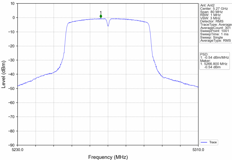
802.11n(HT40)_LCH_5270MHz_MIMO_NTNV
