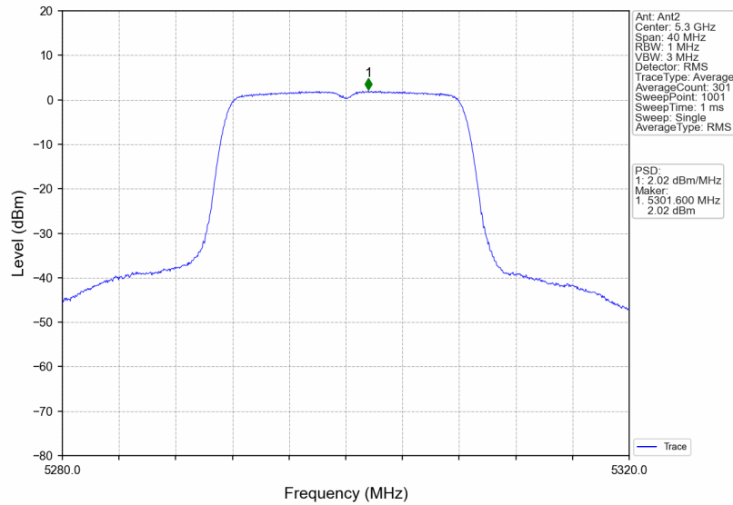
802.11n(HT20)_MCH_5300MHz_MIMO_NTNV
