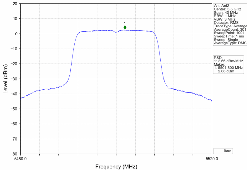
802.11n(HT20)_LCH_5500MHz_MIMO_NTNV
