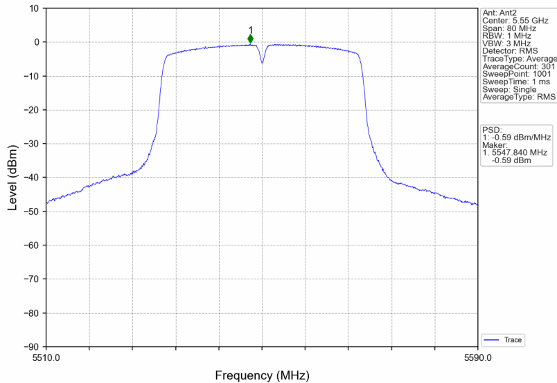
802.11n(HT40)_MCH_5550MHz_MIMO_NTNV
