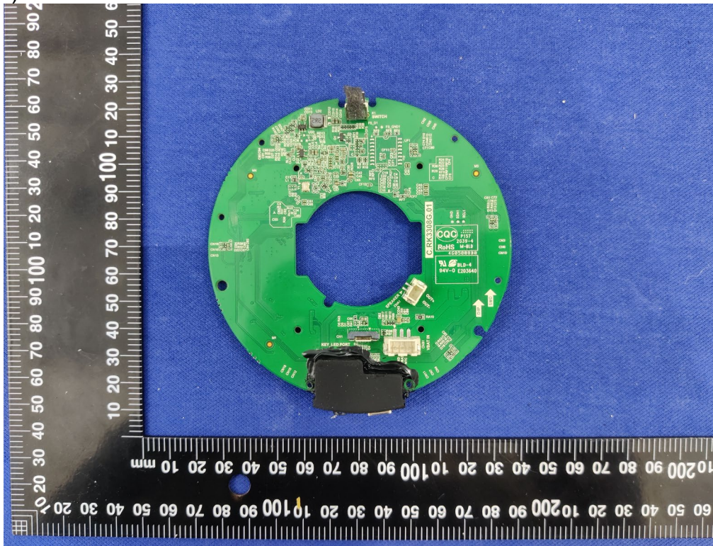
6) EUT Photo
