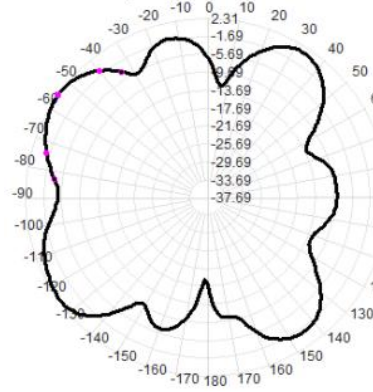
2500.0MHz Total(E1-XZ), Max= 2.31dBi
