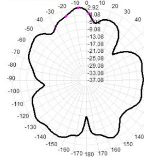
2400.0MHz Total(E2-YZ), Max= 2.92dBi
