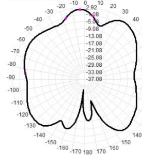
2400.0MHz Total(E1-XZ), Max= 1.77dBi
