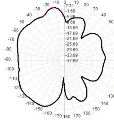
2500.0MHz Total(E2-YZ), Max= 1.65dBi
