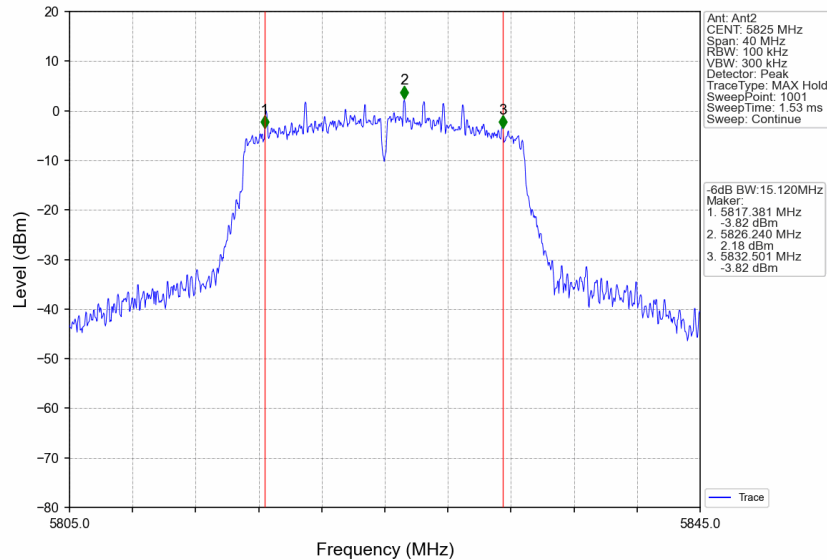
802.11ac(VHT20) HCH 5825MHz Ant2 NTVN
