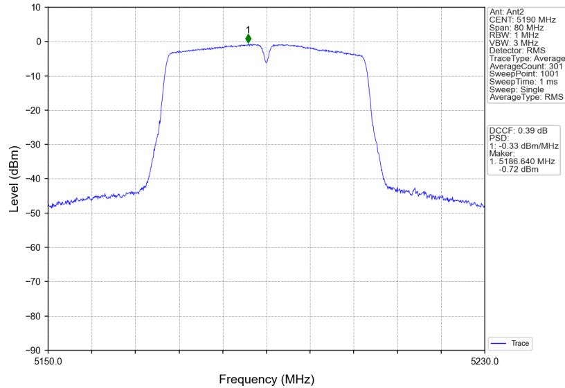
802.11ac(VHT40) LCH 5190MHz MIMO NTV
