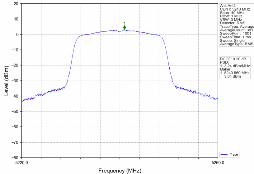
802.11ac(VHT20) HCH 5240MHz Ant2 NTVN
