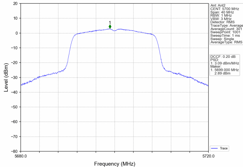
802.11ac(VHT20) HCH 5700MHz Ant2 NTVN
