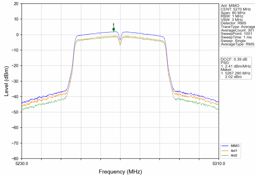
802.11ac(VHT40) LCH 5270MHz MIMO NTV
