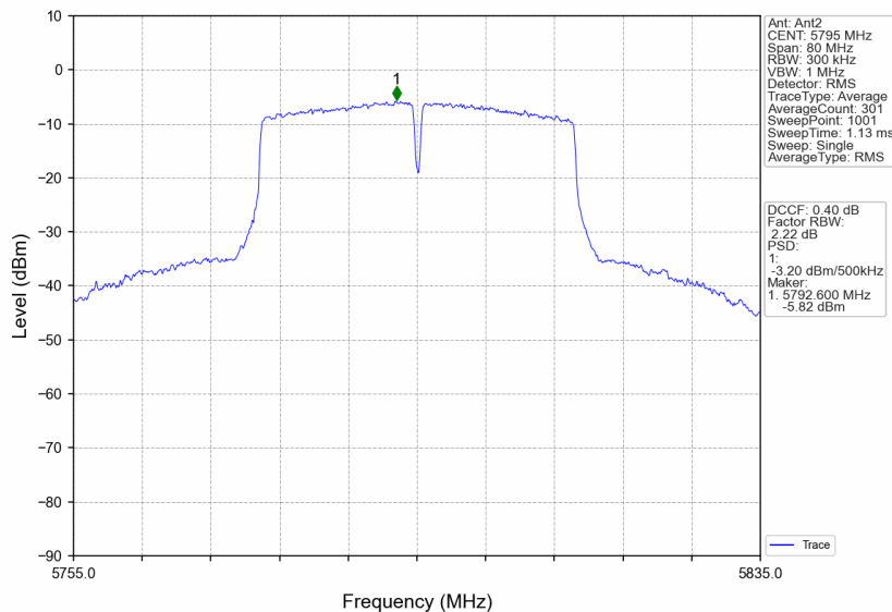
802.11n(HT40) HCH 5795MHz MIMO NTNv
