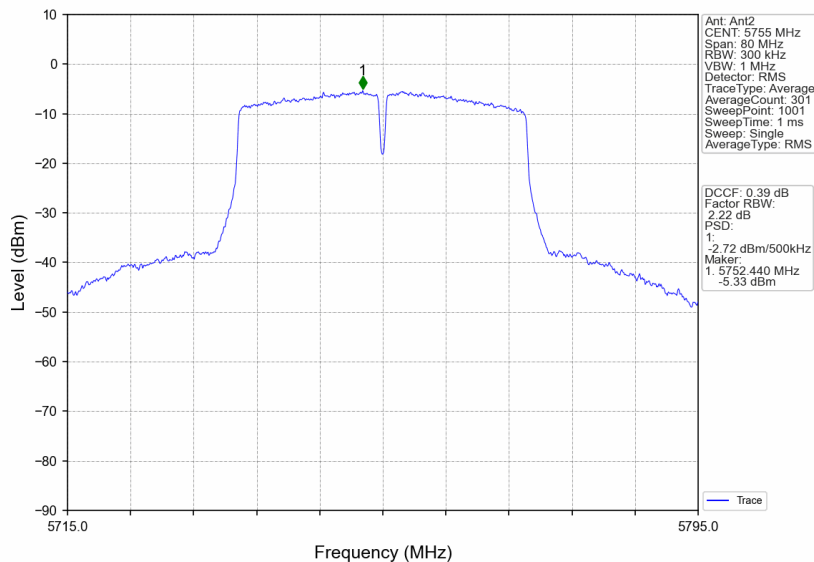
802.11ac(VHT40) LCH 5755MHz MIMO NTNv
