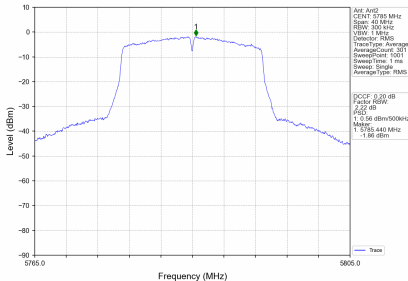
802.11ac(VHT20) MCH 5785MHz MIMO NTNv
