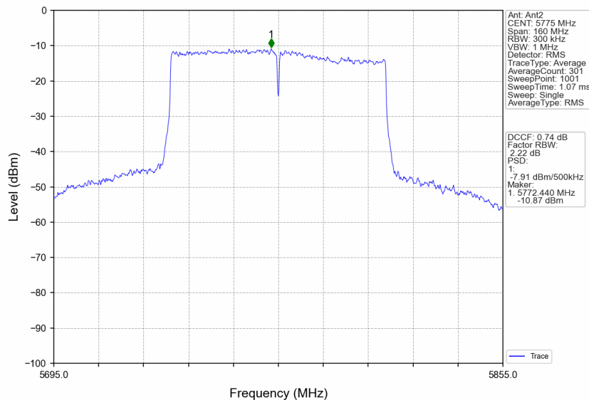
802.11ac(VHT80) MCH 5775MHz MIMO NTNv
