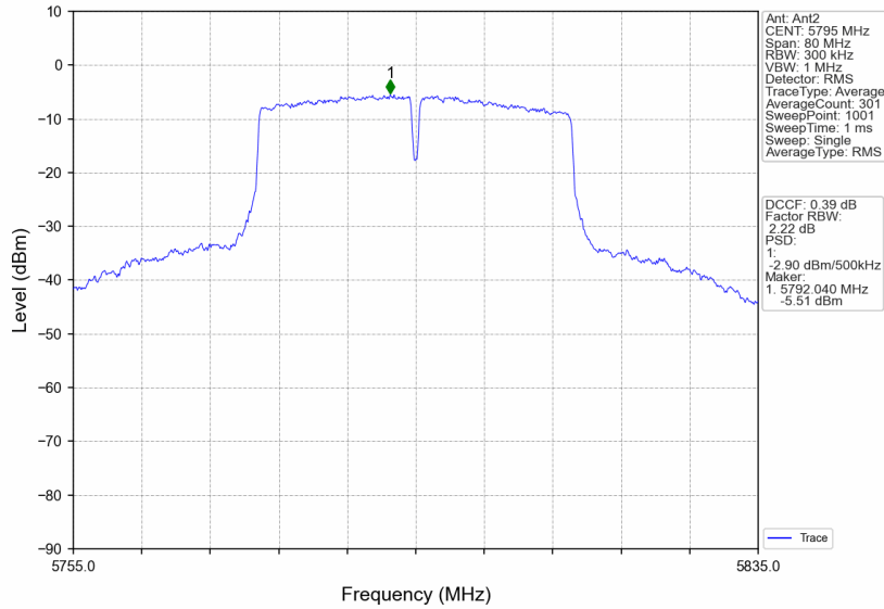
802.11ac(VHT40) HCH 5795MHz MIMO NTN
