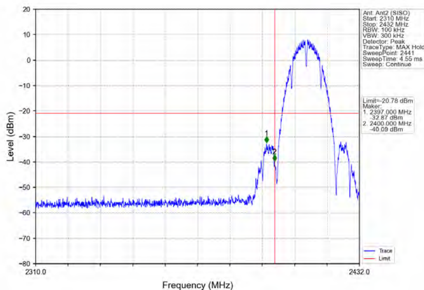
802.11b LCH 2412MHz Ant2 (SISO) NTN
