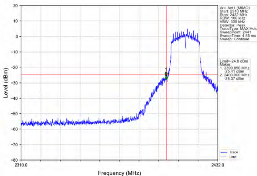
802.11n(HT20) LCH 2412MHz Ant1 (MIMO) NTNV
