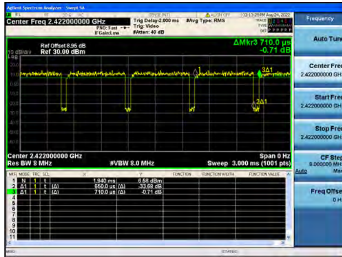
11N40MIMO_Ant2_2422
