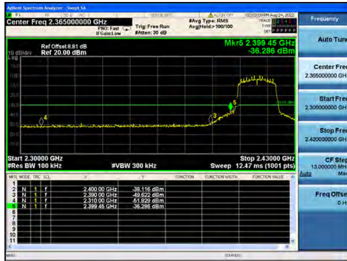
11N20MIMO_Ant2_Low_2412
