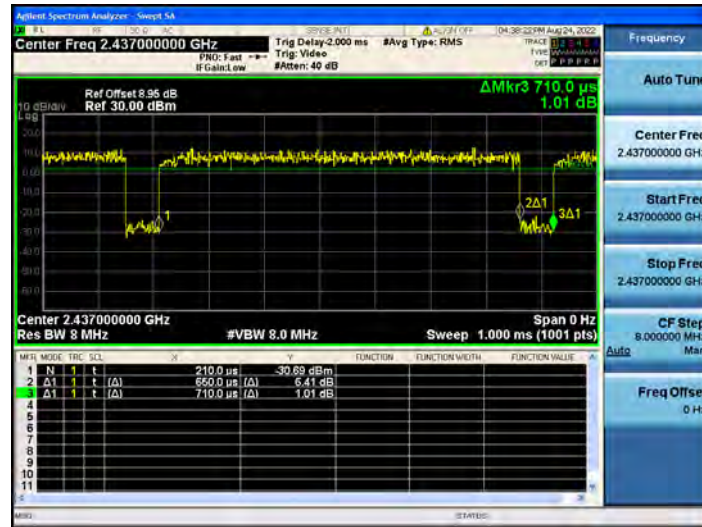
11N40MIMO_Ant2_2437
