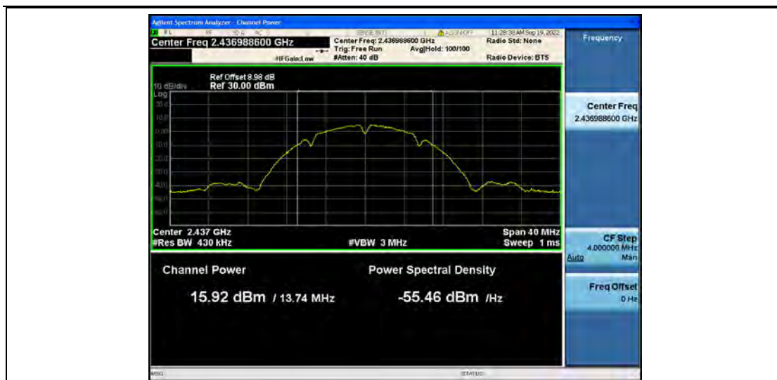
11B_Ant2_2437
