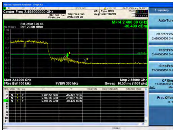
11N40MIMO_Ant2_High_2452
