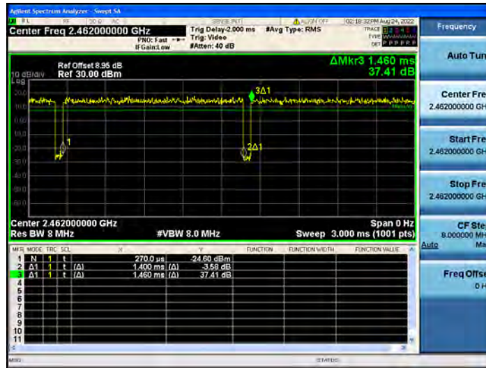
11G_Ant2_2462
