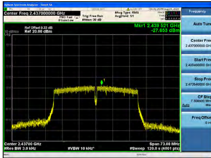
11N40MIMO_Ant2_2437
