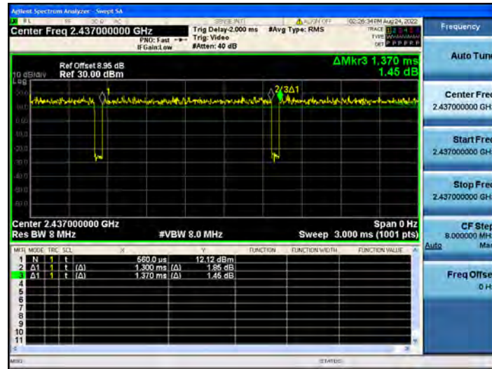
11N20MIMO_Ant2_2437
