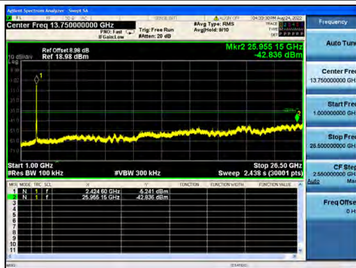
11N40MIMO_Ant1_2437_30~1000
