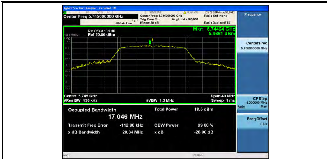
11A_Ant2_5745
