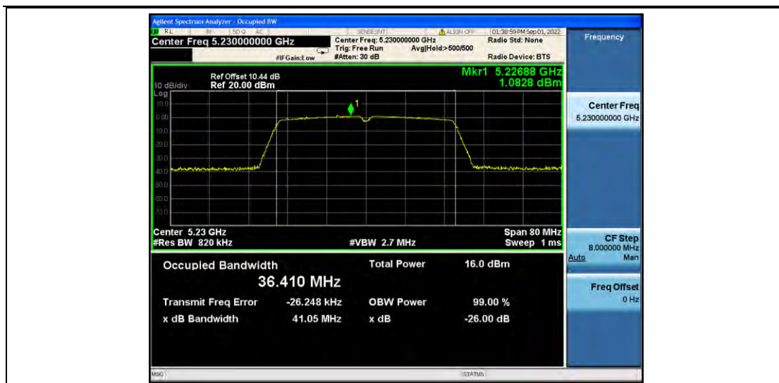
11AC40MIMO_Ant2_5230
