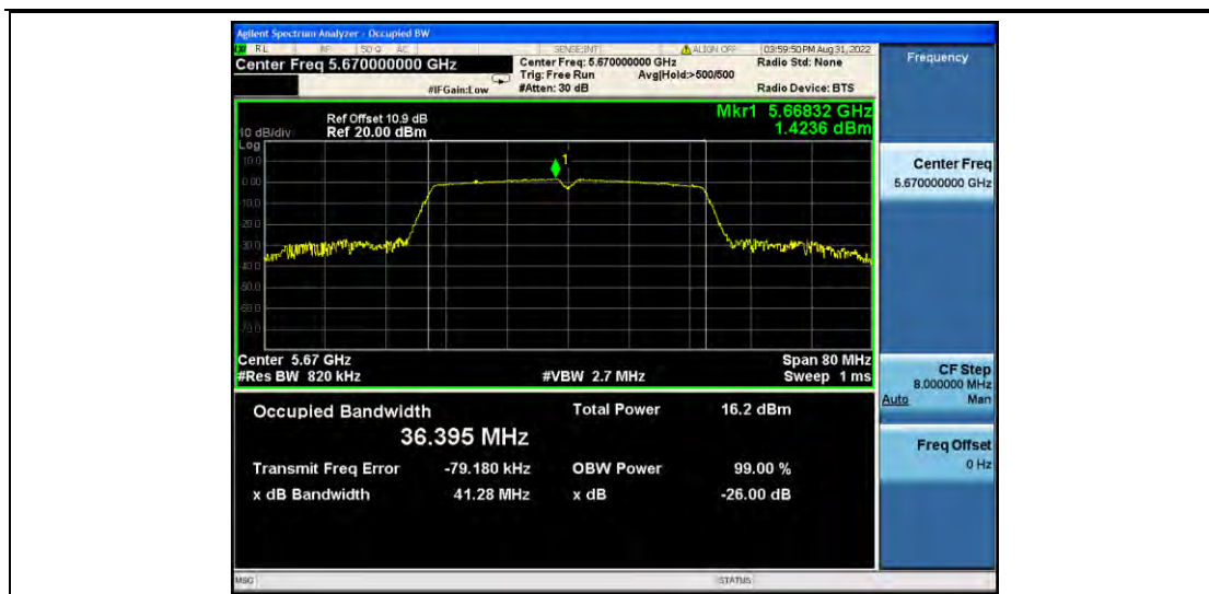
11N40MIMO_Ant2_5670
