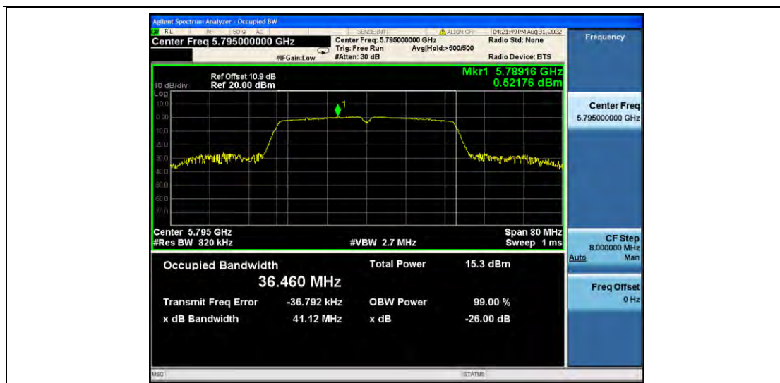
11N40MIMO_Ant2_5795
