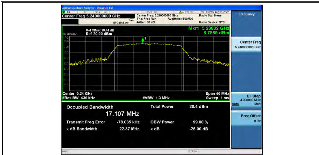
11A_Ant2_5240
