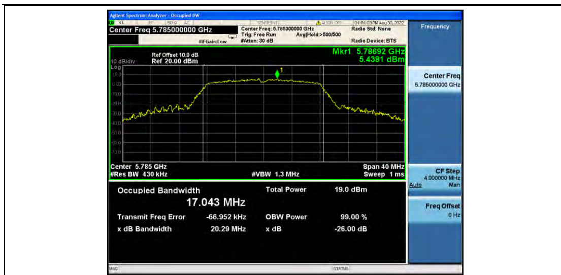
11A_Ant2_5785
