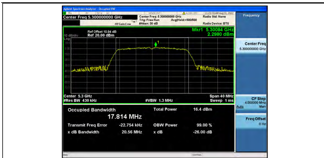
11N20MIMO_Ant2_5300
