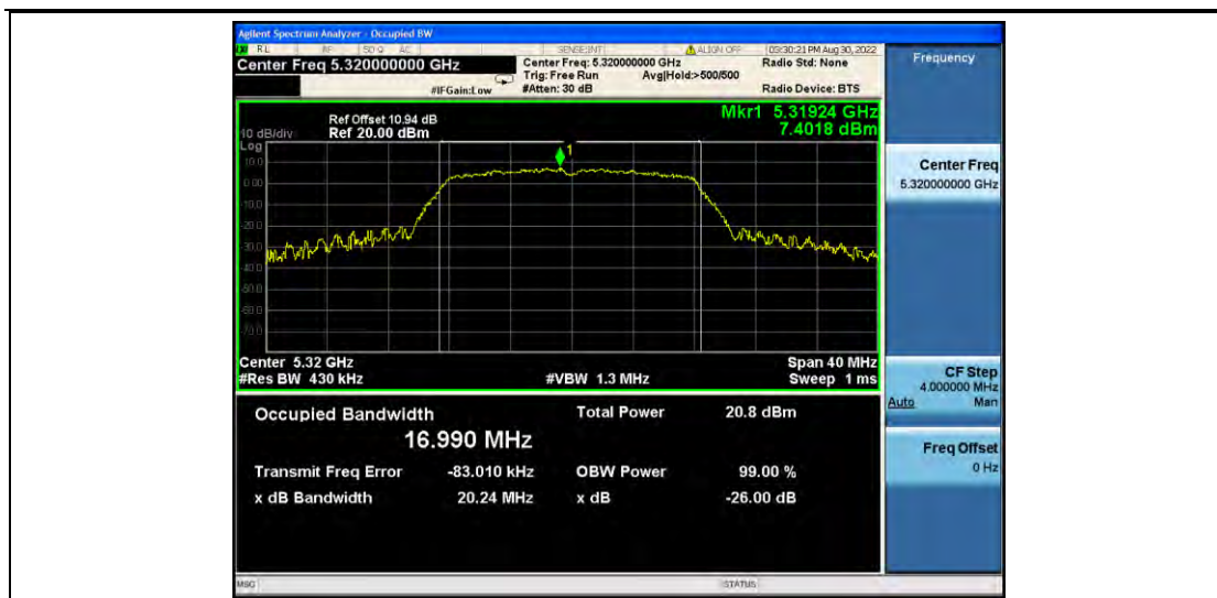
11A_Ant2_5320
