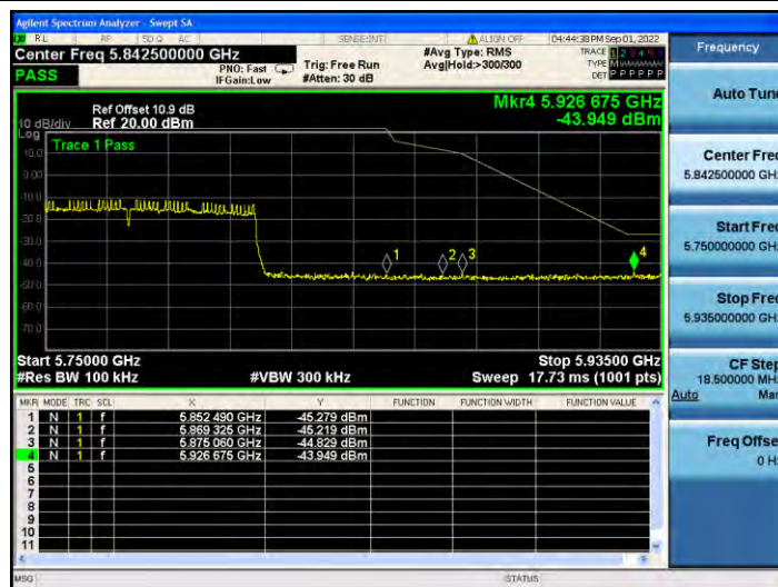
11AC80MIMO_Ant2_Low_5775
