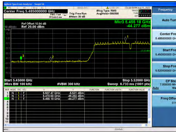
11N40MIMO_Ant2_Low_5510
