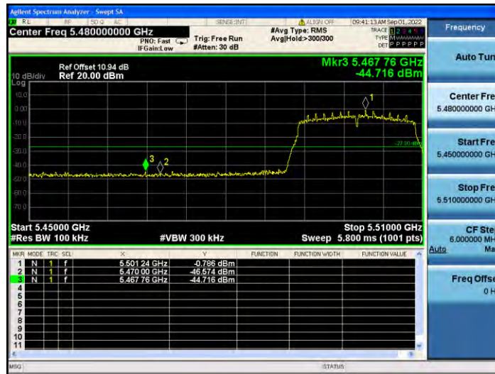
11AC20MIMO_Ant2_Low_5500
