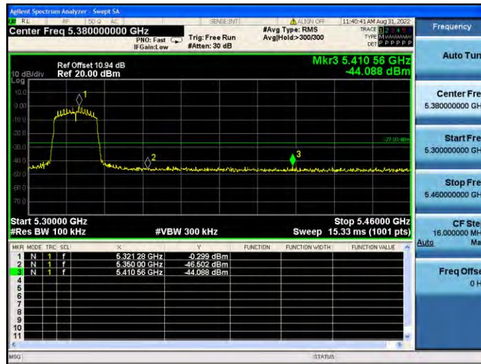
11N20MIMO_Ant2_High_5320
