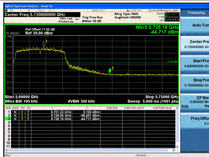
11N40MIMO_Ant1_Low_5190
