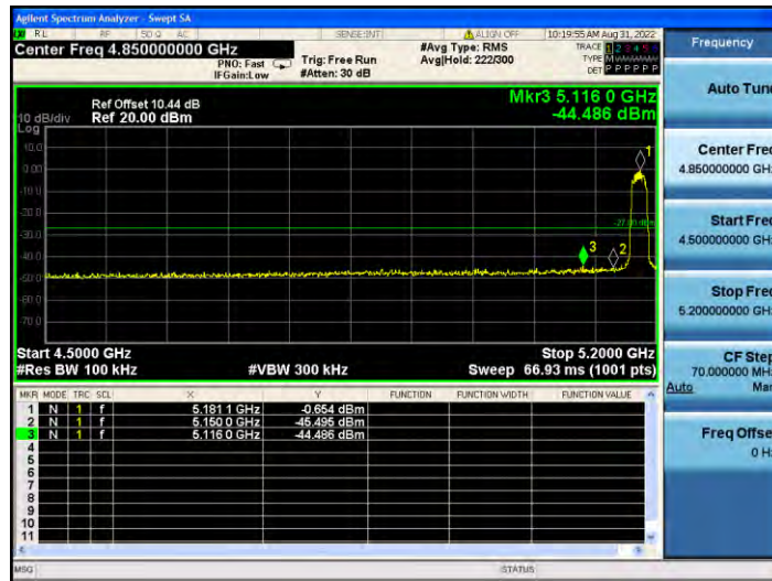
11N20MIMO_Ant2_Low_5180
