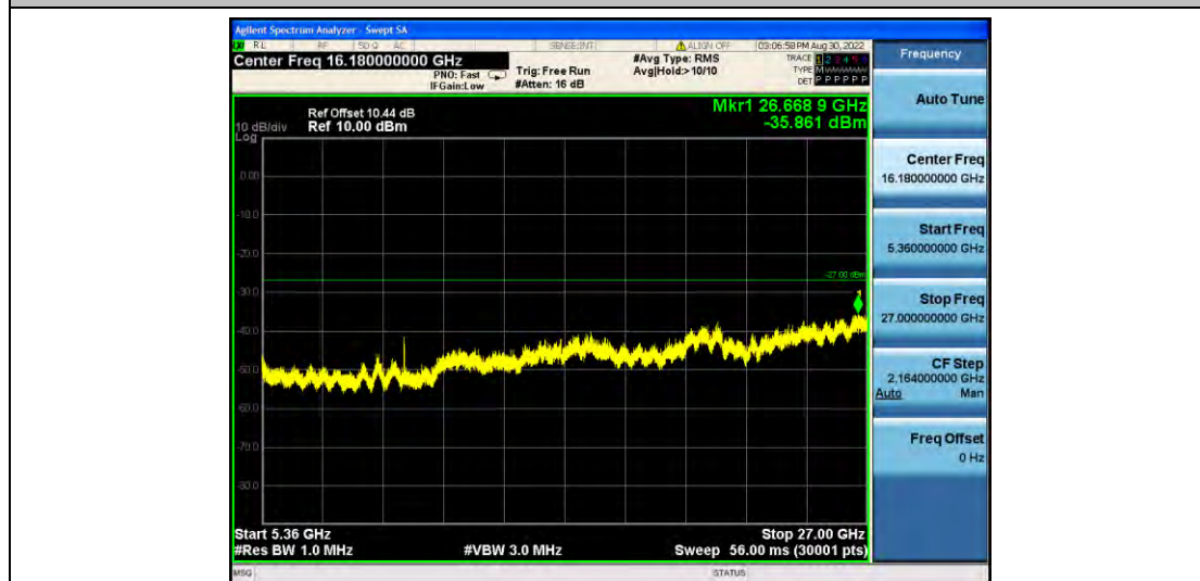
11A_Ant2_5220_30~5140
