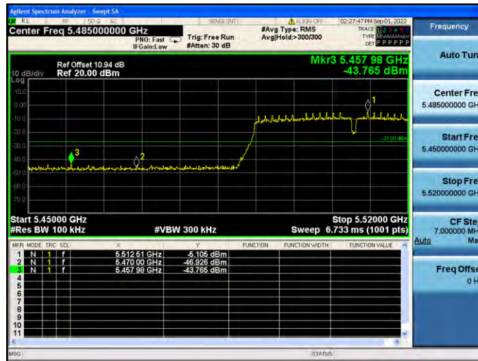
11AC40MIMO_Ant2_Low_5510
