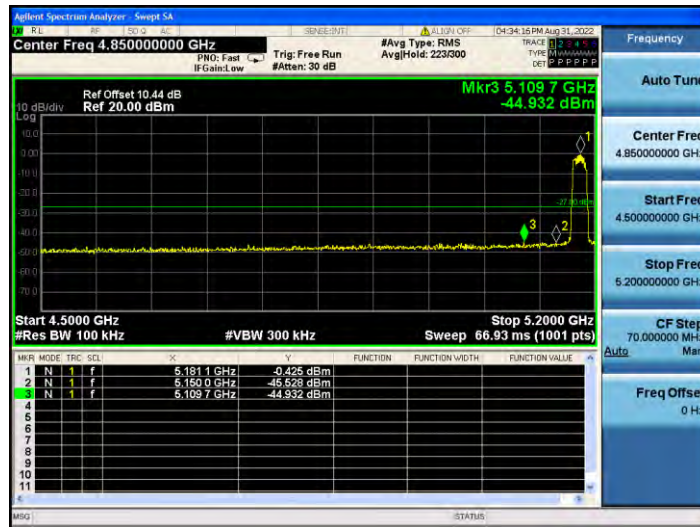
11AC20MIMO_Ant2_Low_5180
