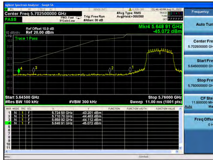
11N20MIMO_Ant2_Low_5745
