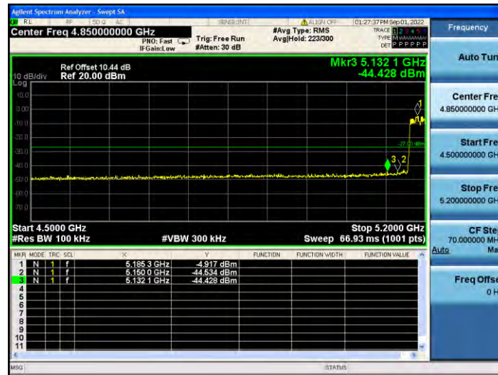
11AC40MIMO_Ant2_Low_5190
