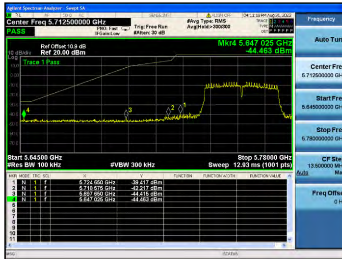
11N40MIMO_Ant2_Low_5755
