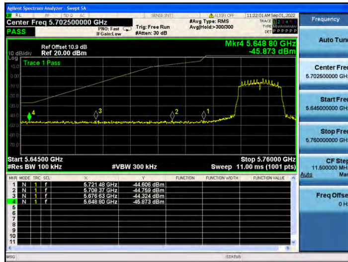
11AC20MIMO_Ant2_Low_5745
