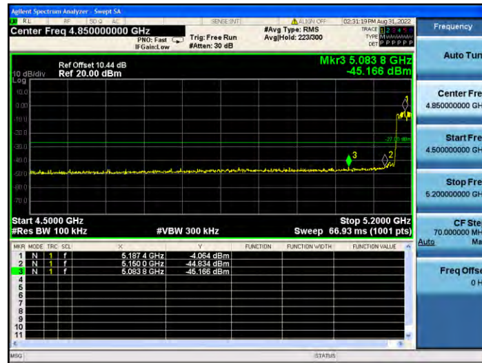
11N40MIMO_Ant2_Low_5190
