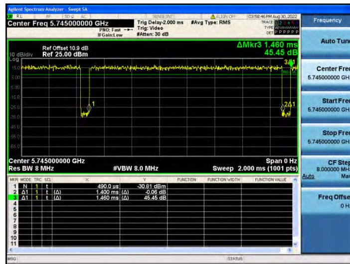
11A_Ant2_5745
