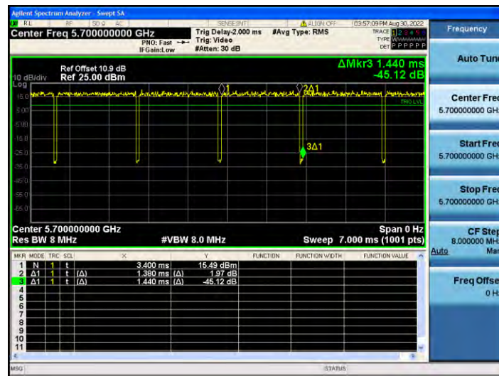
11A_Ant2_5700
