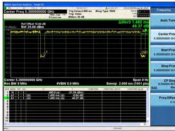
11A_Ant2_5300
