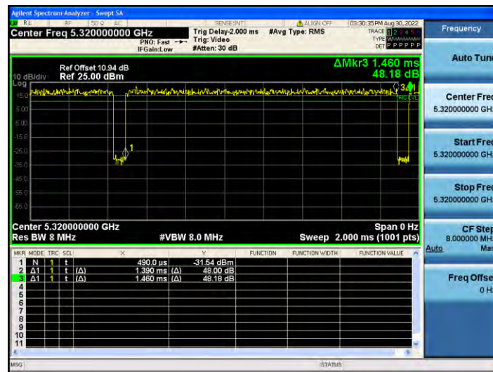
11A_Ant2_5320
