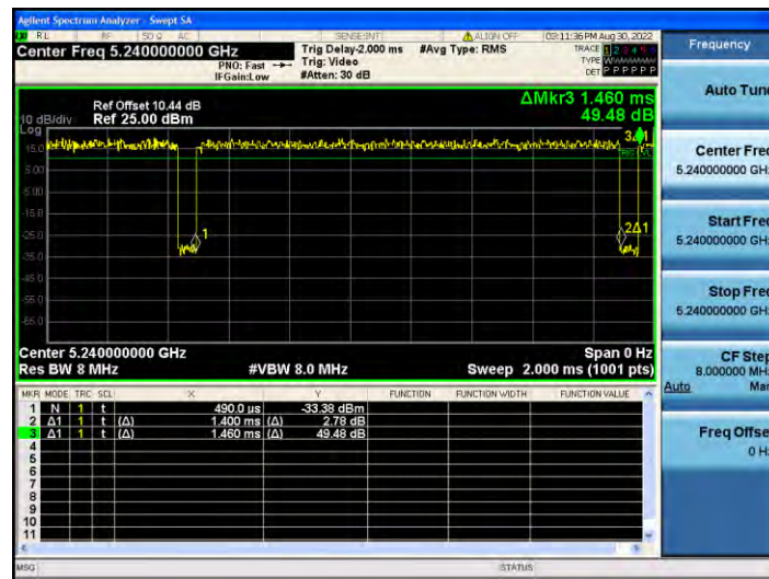
11A_Ant2_5240
