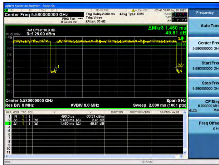
11A_Ant2_5580
