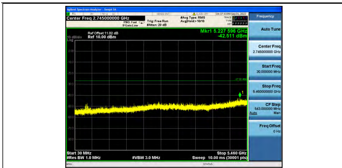
11AC80MIMO_Ant2_5610_5735~40000
