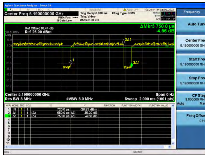
11AC40MIMO_Ant2_5190
