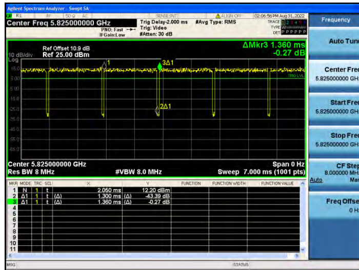
11N20MIMO_Ant2_5825
