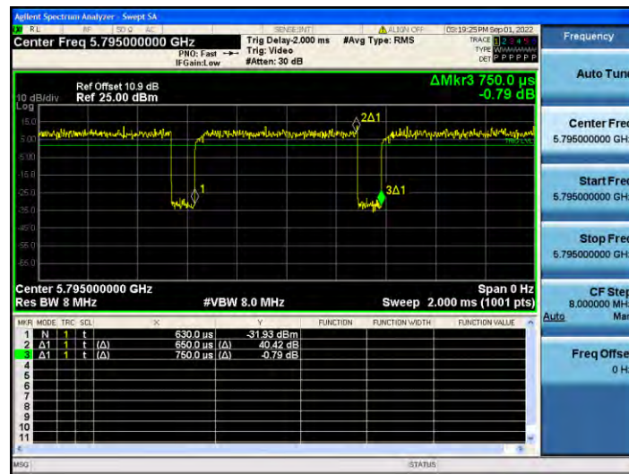
11AC40MIMO_Ant2_5795
