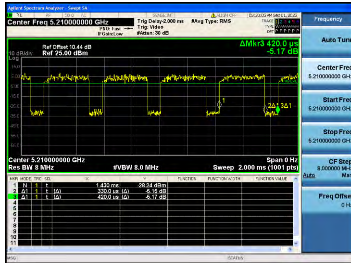
11AC80MIMO_Ant2_5210
