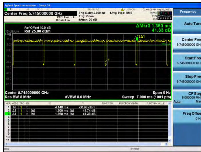
11N20MIMO_Ant2_5745
