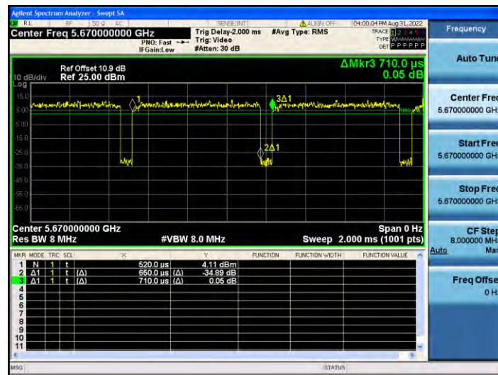
11N40MIMO_Ant2_5670
