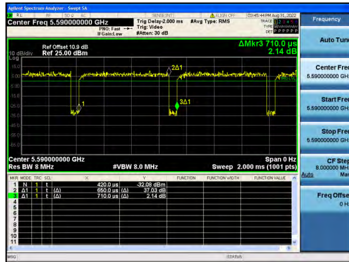
11N40MIMO_Ant2_5590
