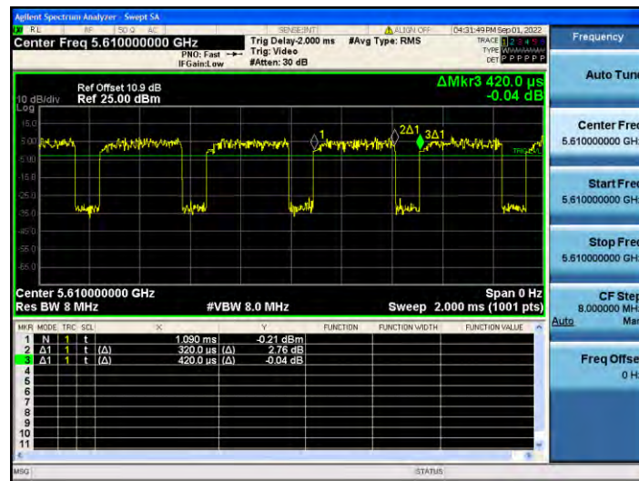
11AC80MIMO_Ant2_5610
