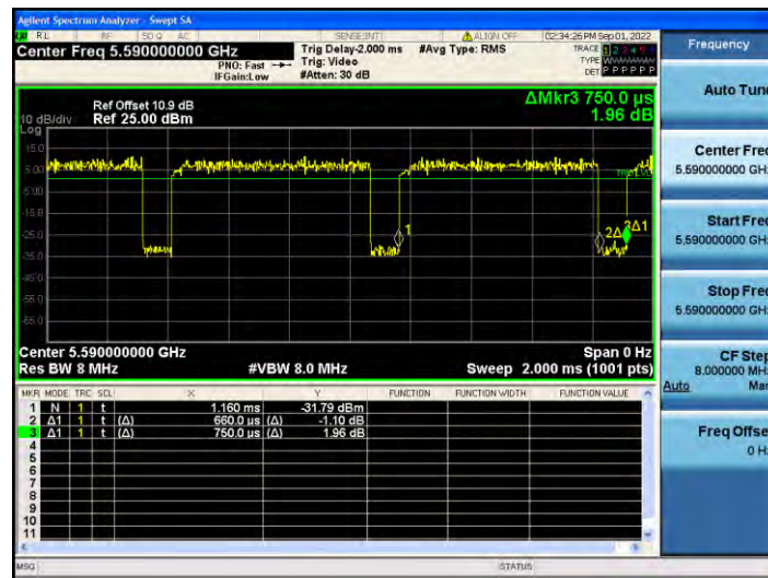
11AC40MIMO_Ant2_5590
