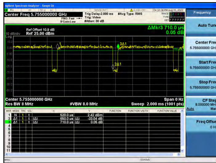
11N40MIMO_Ant2_5755
