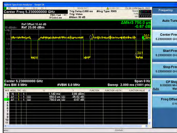
11AC40MIMO_Ant2_5230
