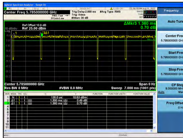
11N20MIMO_Ant2_5785
