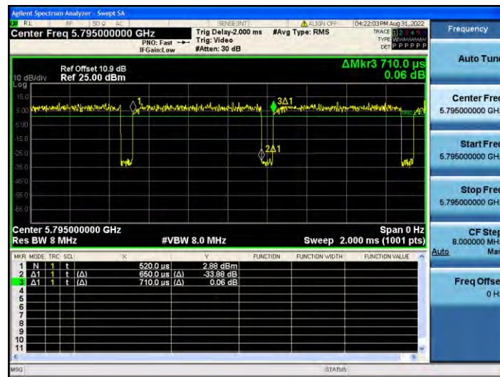
11N40MIMO_Ant2_5795
