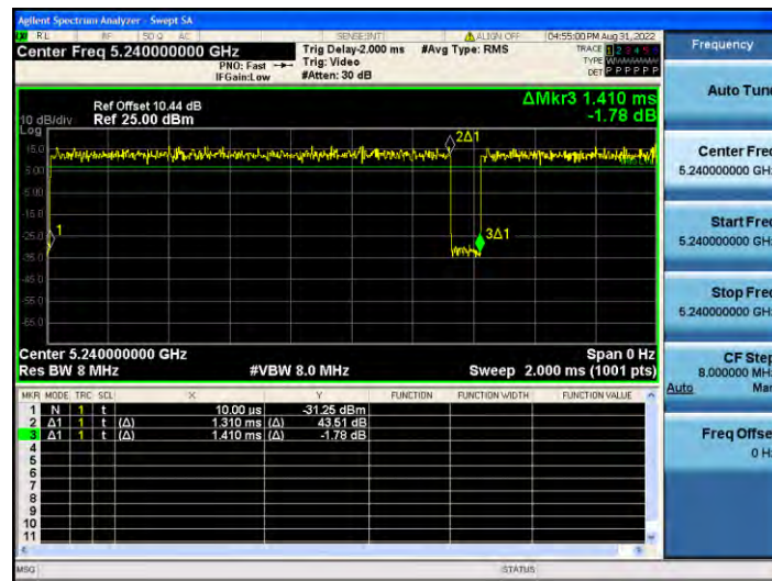
11AC20MIMO_Ant2_5240
