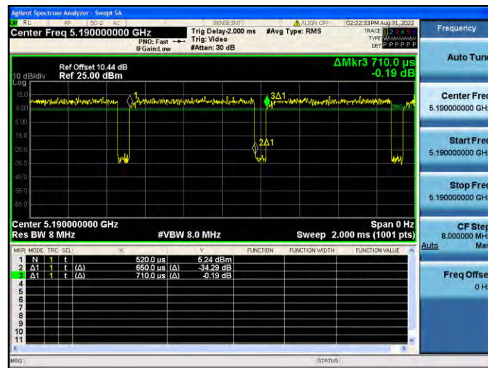
11N40MIMO_Ant2_5190
