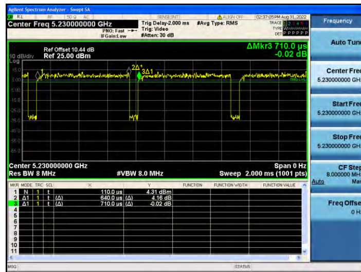
11N40MIMO_Ant2_5230
