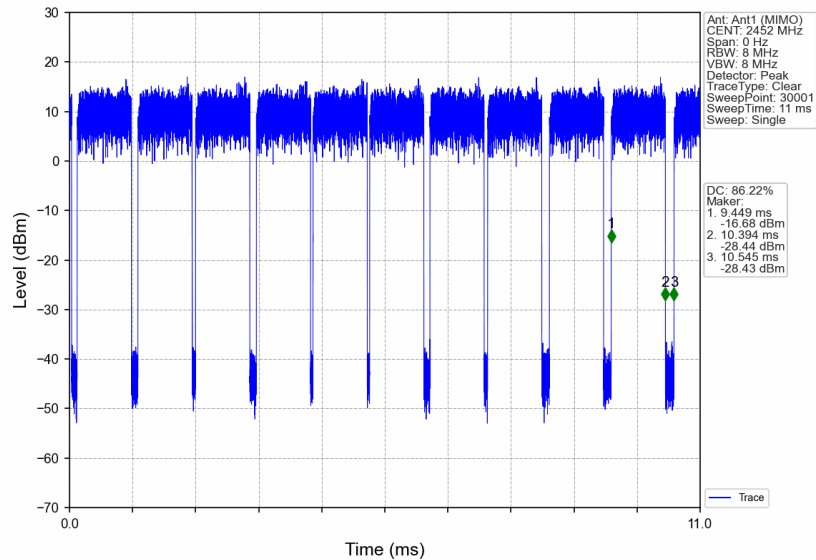
802.11n(HT40) HCH 2452MHz Ant1 (MIMO) NTVN
