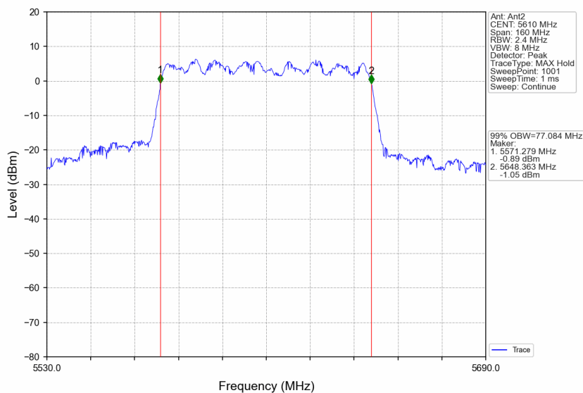
802.11ac(VHT80)_HCH_5610MHz_Ant2_NTNV
