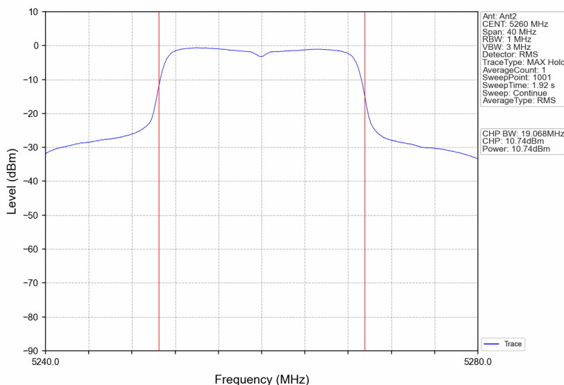
802.11n(HT20)_LCH_5260MHz_Ant2_NTNV
