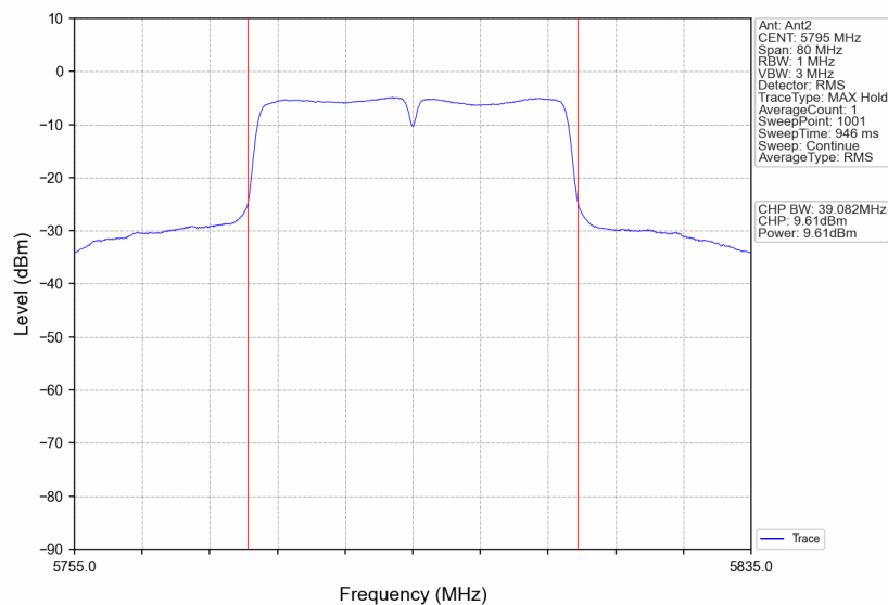
802.11n(HT40)_HCH_5795MHz_Ant2_NTNV
