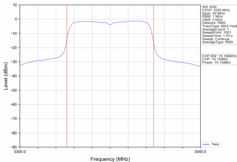
802.11n(HT20)_HCH_5320MHz_Ant2_NTNV
