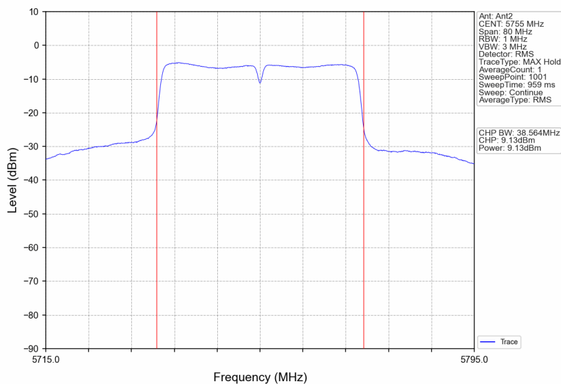
802.11ac(VHT40)_LCH_5755MHz_Ant2_NTNV
