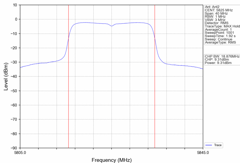
802.11n(HT20)_HCH_5825MHz_Ant2_NTNV
