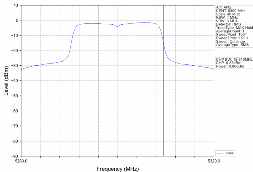
802.11n(HT20)_MCH_5300MHz_Ant2_NTNV
