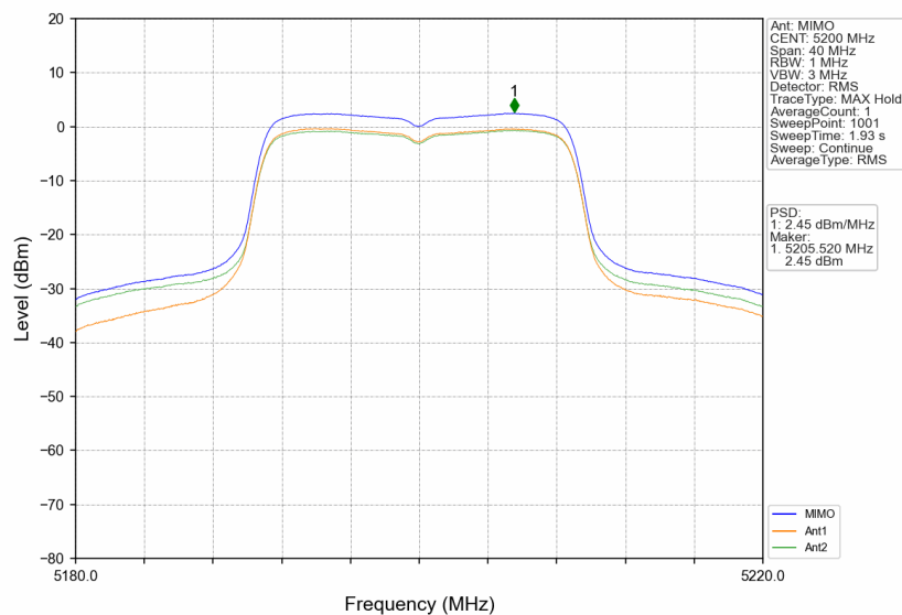
802.11n(HT20)_MCH_5200MHz_MIMO_NTNV
