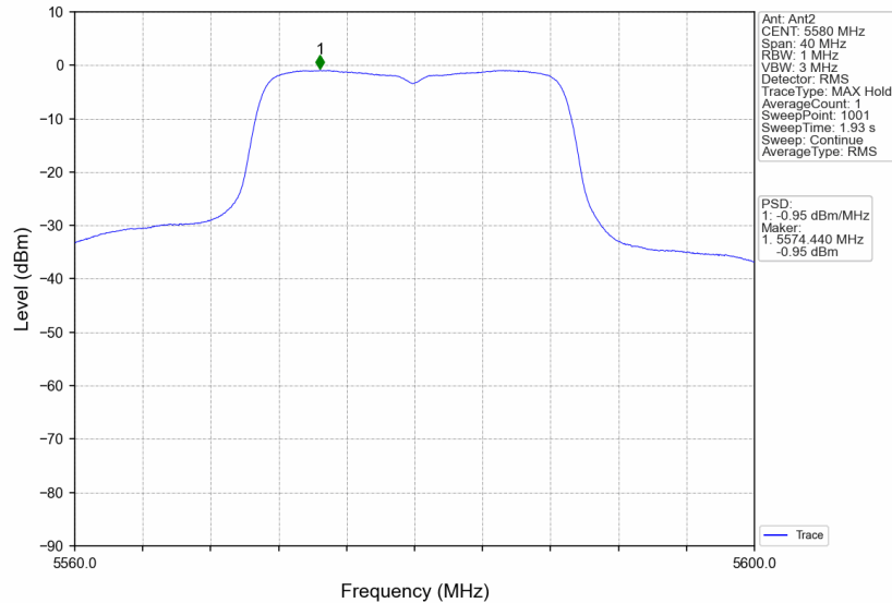
802.11n(HT20)_MCH_5580MHz_MIMO_NTNV
