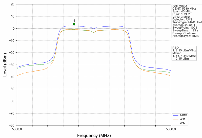
802.11n(HT20)_MCH_5580MHz_MIMO_NTNV
