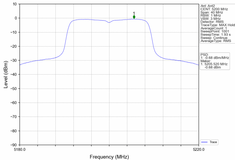
802.11n(HT20)_MCH_5200MHz_MIMO_NTNV
