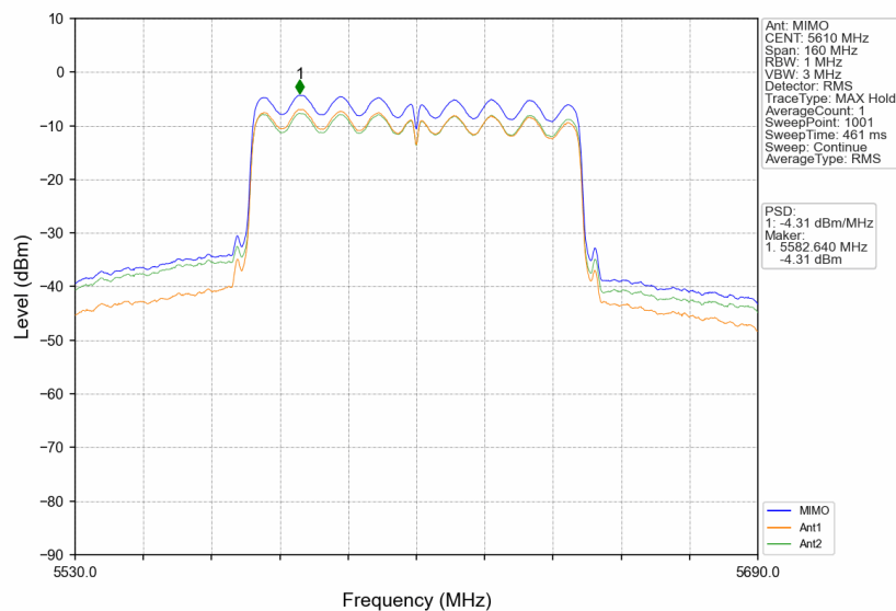
802.11ac(VHT80)_HCH_5610MHz_MIMO_NTNV
