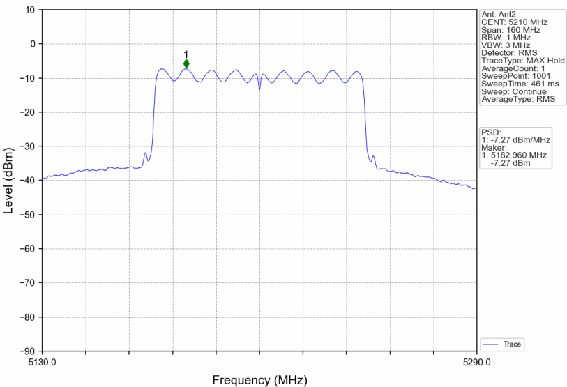
802.11ac(VHT80)_MCH_5210MHz_Ant2_NTNV
