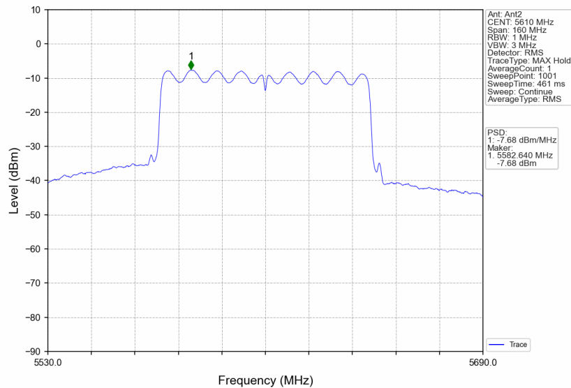
802.11ac(VHT80)_HCH_5610MHz_MIMO_NTNV
