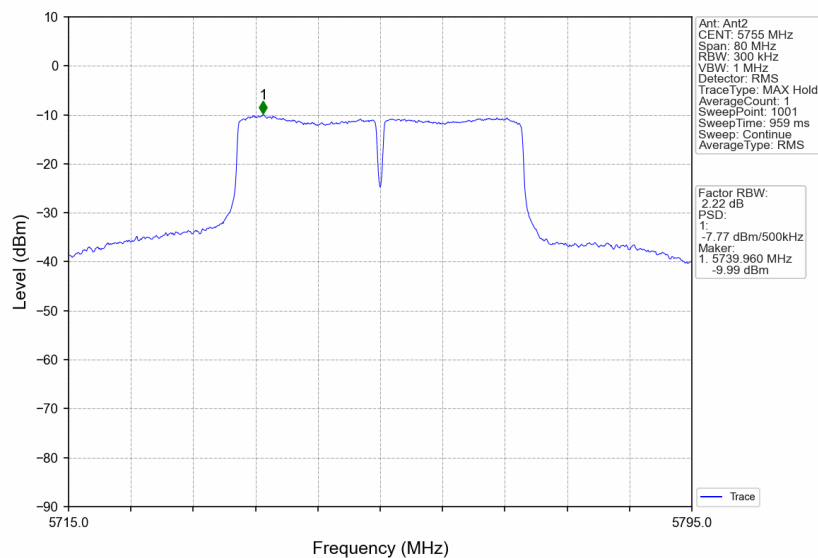
802.11ac(VHT40)_LCH_5755MHz_Ant2_NTNV
