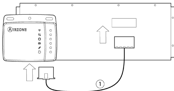
Anschlusschema
