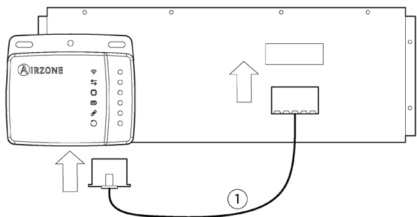
Esquema de conexión orientativo
