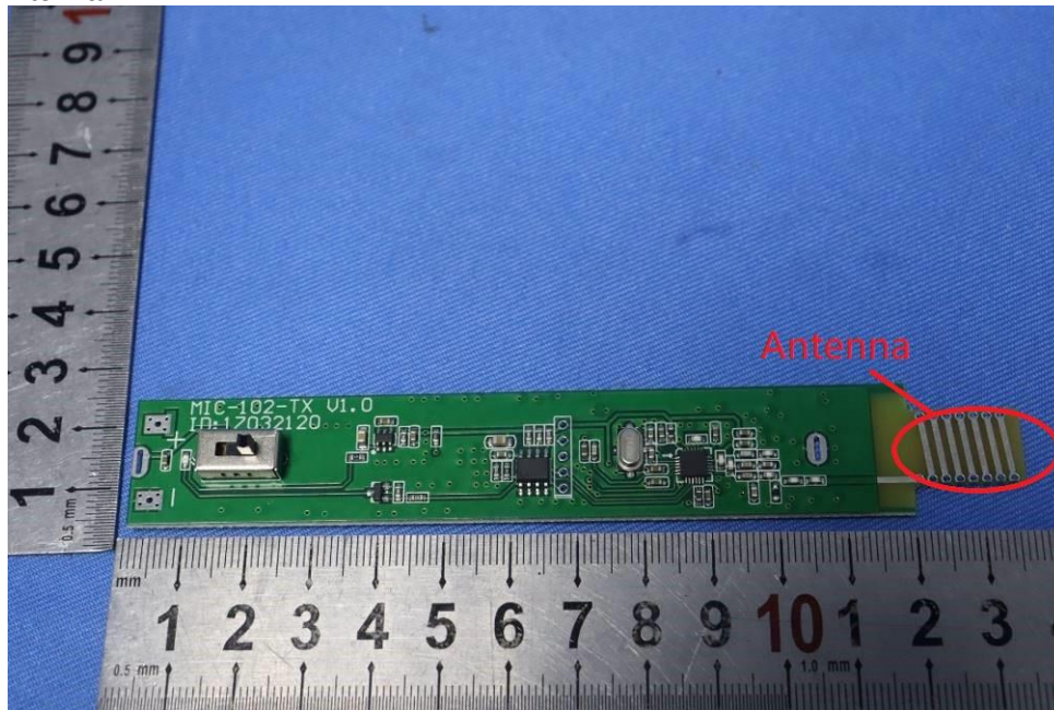
Antenna
