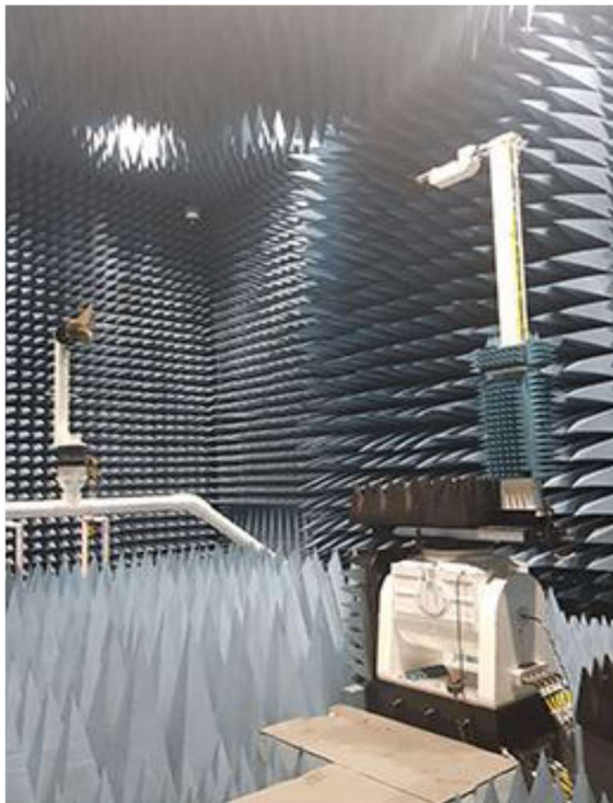
Anechoic Chamber(AMS-8500)
