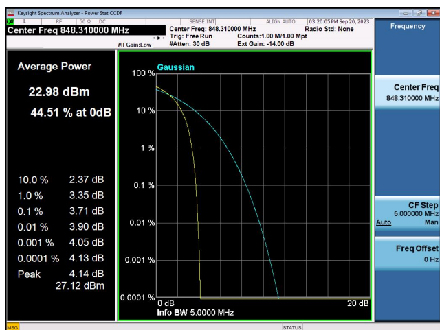
CDMA2000 BC0-777
