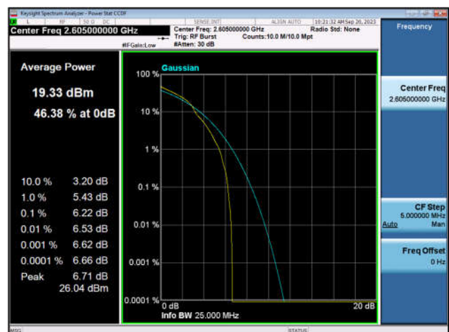
TDD41_MidRange_20MHz_2605_OneRB_high_Q16
