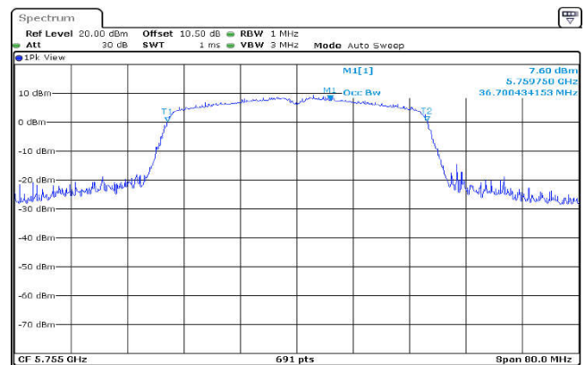
U-NII-3,802.11ac(40MHz),5755MHz ,Ant1
