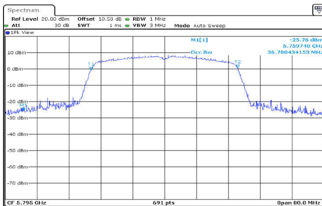
U-NII-3,802.11ac(40MHz),5795MHz ,Ant1
