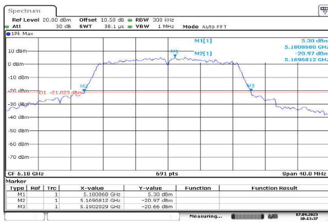
U-NII-1,802.11n(20MHz),5180MHz ,Ant1
