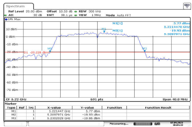
U-NII-1,802.11n(20MHz),5220MHz ,Ant1
