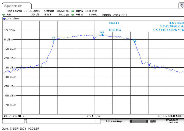
U-NII-1,802.11ac(20MHz),5240MHz ,Ant1
