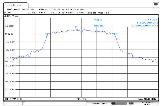
U-NII-1,802.11n(20MHz),5220MHz ,Ant1
