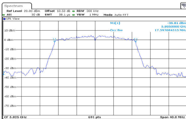
U-NII-3,802.11ac(20MHz),5825MHz ,Ant1
