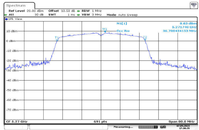
U-NII-2a,802.11ac(40MHz),5270MHz ,Ant1
